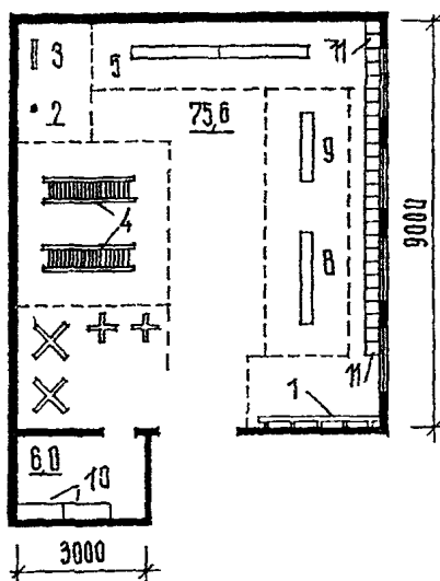
Рис. 40 Расстановка оборудования в залах для музыкальных и физкультурных занятий а - для физкультурных занятий площадью 100 м 2 ; б - то же, площадью 75 м 2 ; в - для музыкальных занятий 1 - стенка гимнастическая; 2 - канат; 3 - кольцо для пролезания; 4 - мостик-качалка; 5 - скамья гимнастическая; 6 - стойка для игровых пособий; 7 - стойка для прыжков; 8 - бревно гимнастическое; 9 - бревно круглое; 10 - шкаф для спортивного инвентаря; 11 - стул детский; 12 - пианино; 13 - табурет для пианино; 14 - шкаф для пособий
