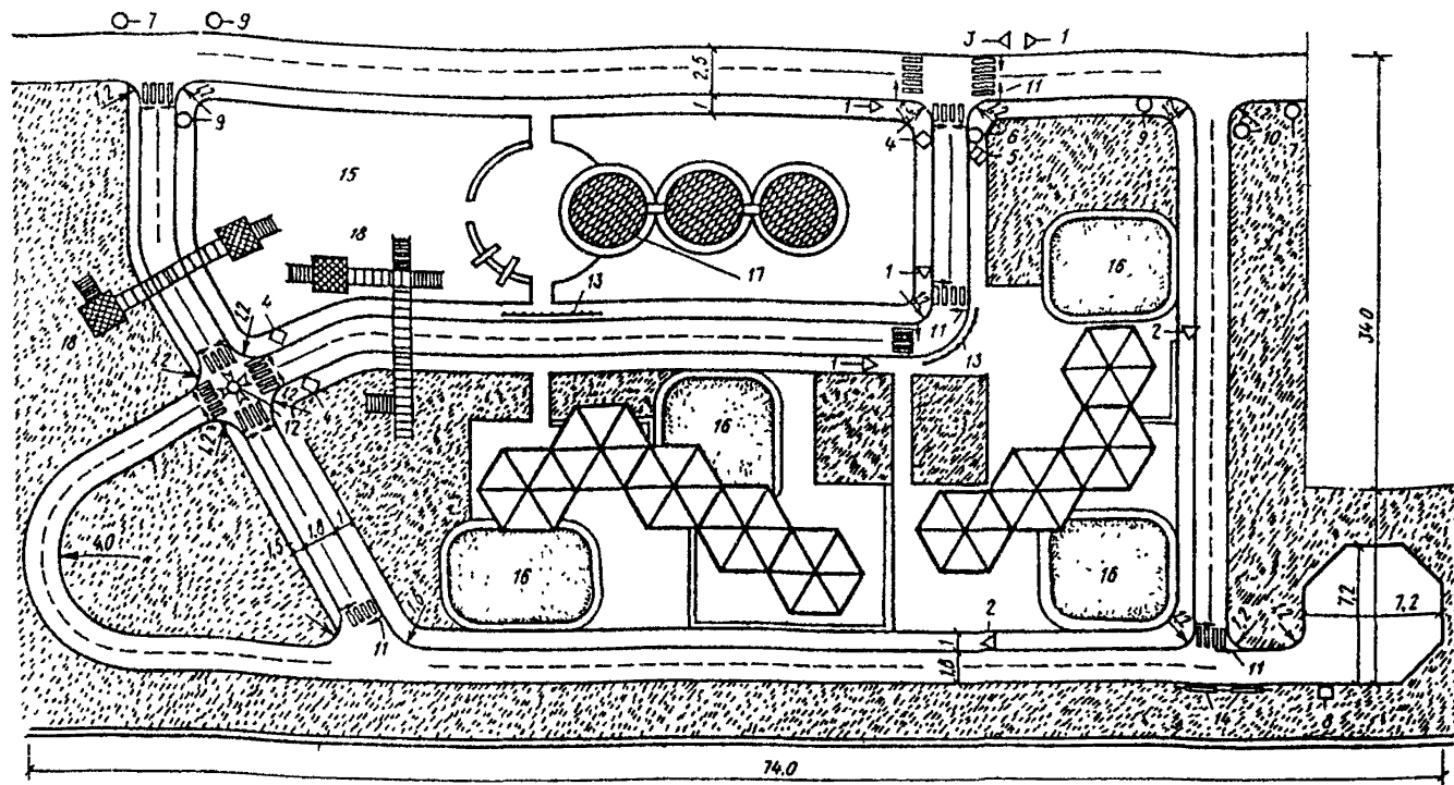
Рис. 10 Пример планировки и оборудования площадки для обучения детей правилам дорожного движения
