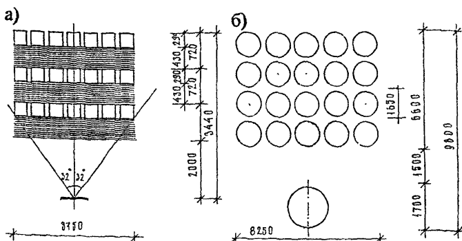
Рис. 39 Габариты отдельных функциональных зон в зале для музыкальных и гимнастических занятий
