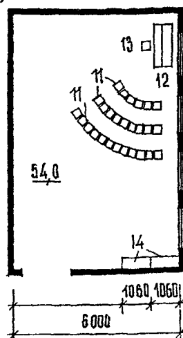
Рис. 40 Расстановка оборудования в залах для музыкальных и физкультурных занятий а - для физкультурных занятий площадью 100 м 2 ; б - то же, площадью 75 м 2 ; в - для музыкальных занятий 1 - стенка гимнастическая; 2 - канат; 3 - кольцо для пролезания; 4 - мостик-качалка; 5 - скамья гимнастическая; 6 - стойка для игровых пособий; 7 - стойка для прыжков; 8 - бревно гимнастическое; 9 - бревно круглое; 10 - шкаф для спортивного инвентаря; 11 - стул детский; 12 - пианино; 13 - табурет для пианино; 14 - шкаф для пособий
