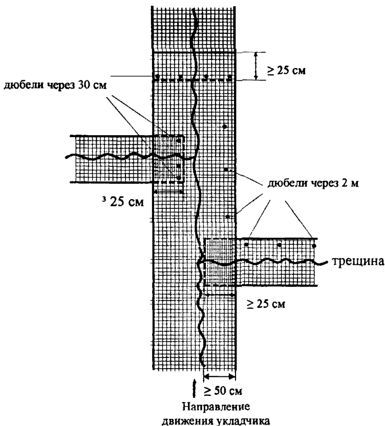
Рисунок 1 – Схема расположения полотен геосеток при локальном армировании
