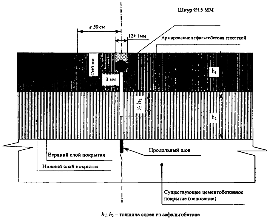
Рисунок 3 – Схема конструкции шва и расположение армирующей прослойки при локальном армировании продольного шва (поперечное сечение)
