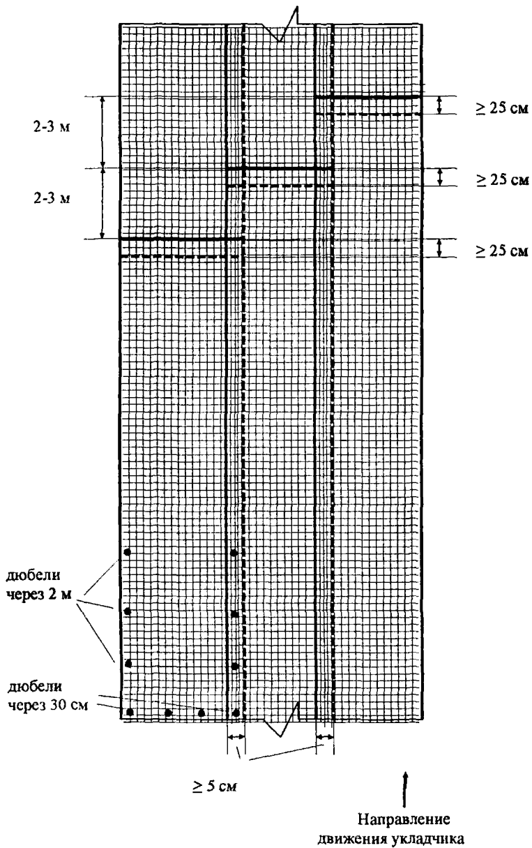
Рисунок 2 – Схема расположения полотен геосеток при сплошном армировании
