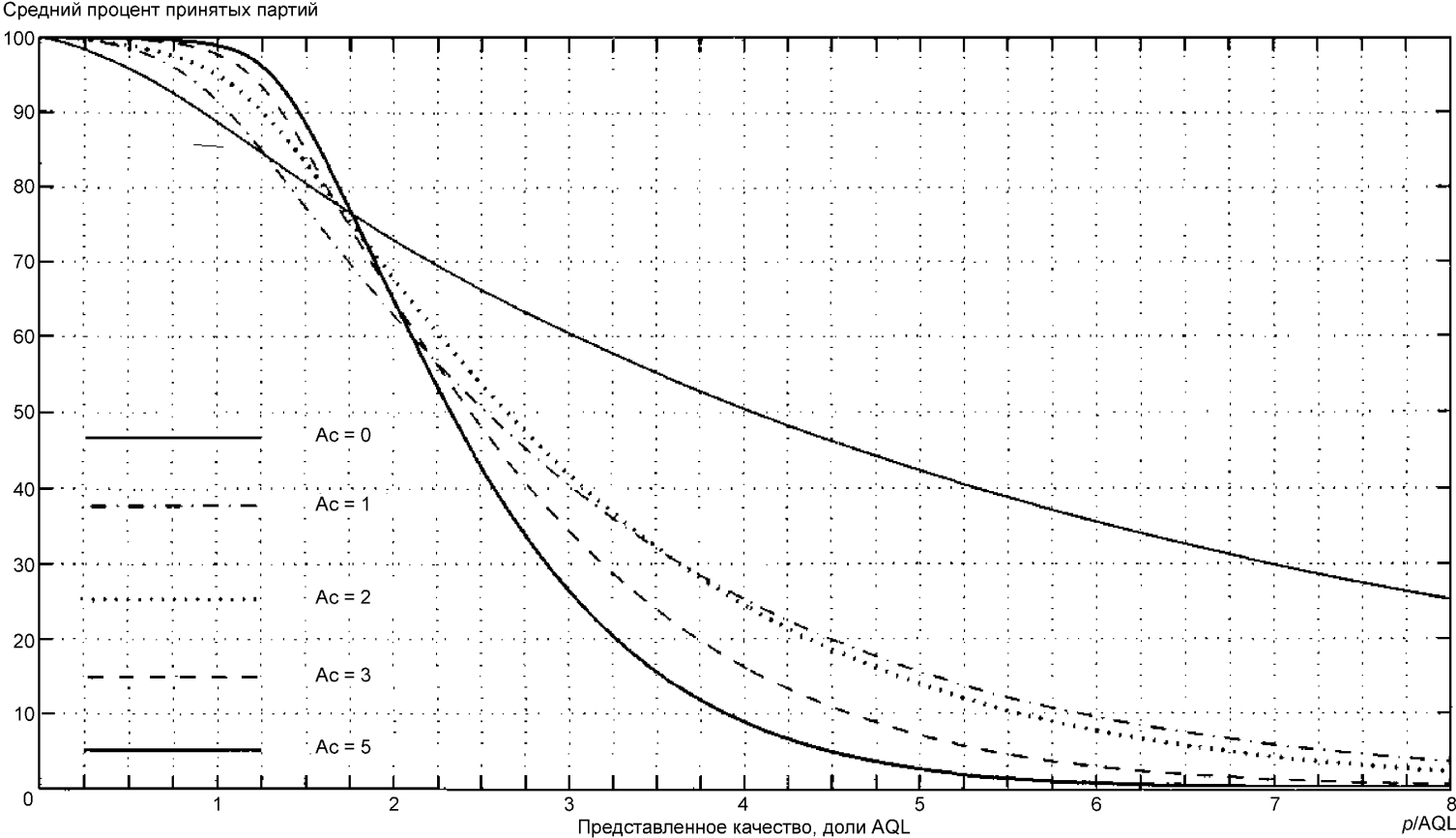
96 Таблица 12 — График нормализованных кривых оперативных характеристик
