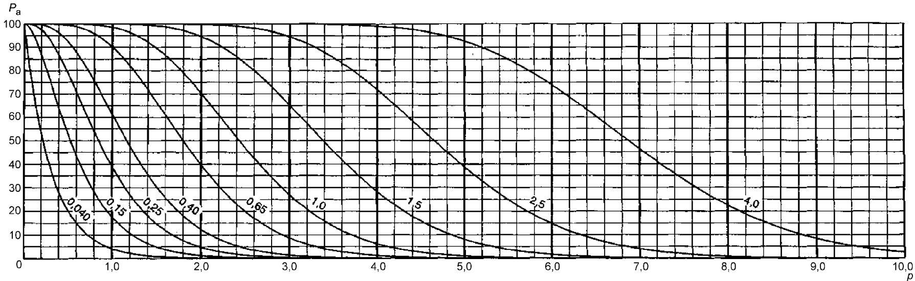
График М — Кривые оперативных характеристик для одноступенчатых планов (кривые для двухступенчатого и многоступенчатого планов контроля максимально близки)
