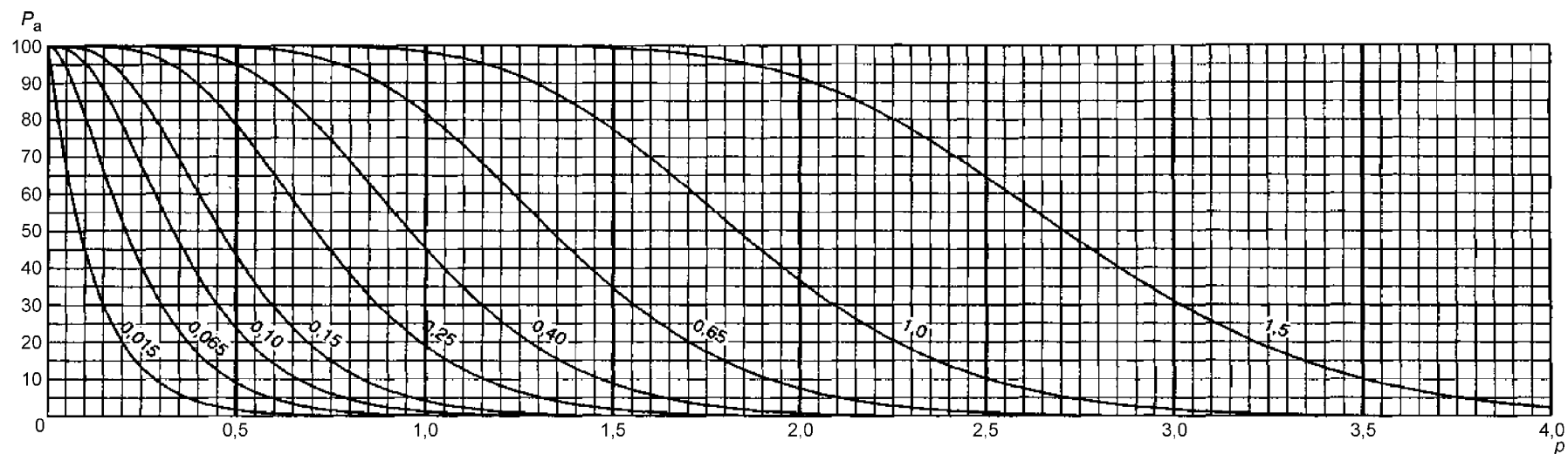
График Р — Кривые оперативных характеристик для одноступенчатых планов (кривые для двухступенчатого и многоступенчатого планов контроля максимально близки)
