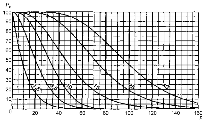
График D — Кривые оперативных характеристик для одноступенчатых планов (кривые для двухступенчатого и многоступенчатого планов контроля максимально близки)
