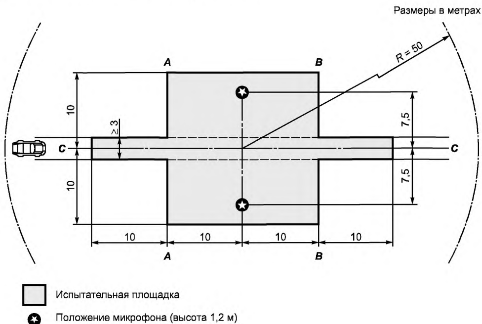
Рисунок 1 — Размеры испытательной площадки
