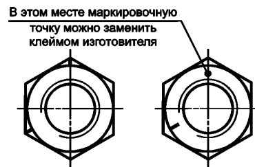
Рисунок 4 — Примеры маркировки кодовым символом (система циферблата)
