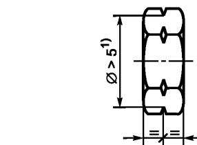
Рисунок 6 — Альтернативная маркировка левой резьбы
