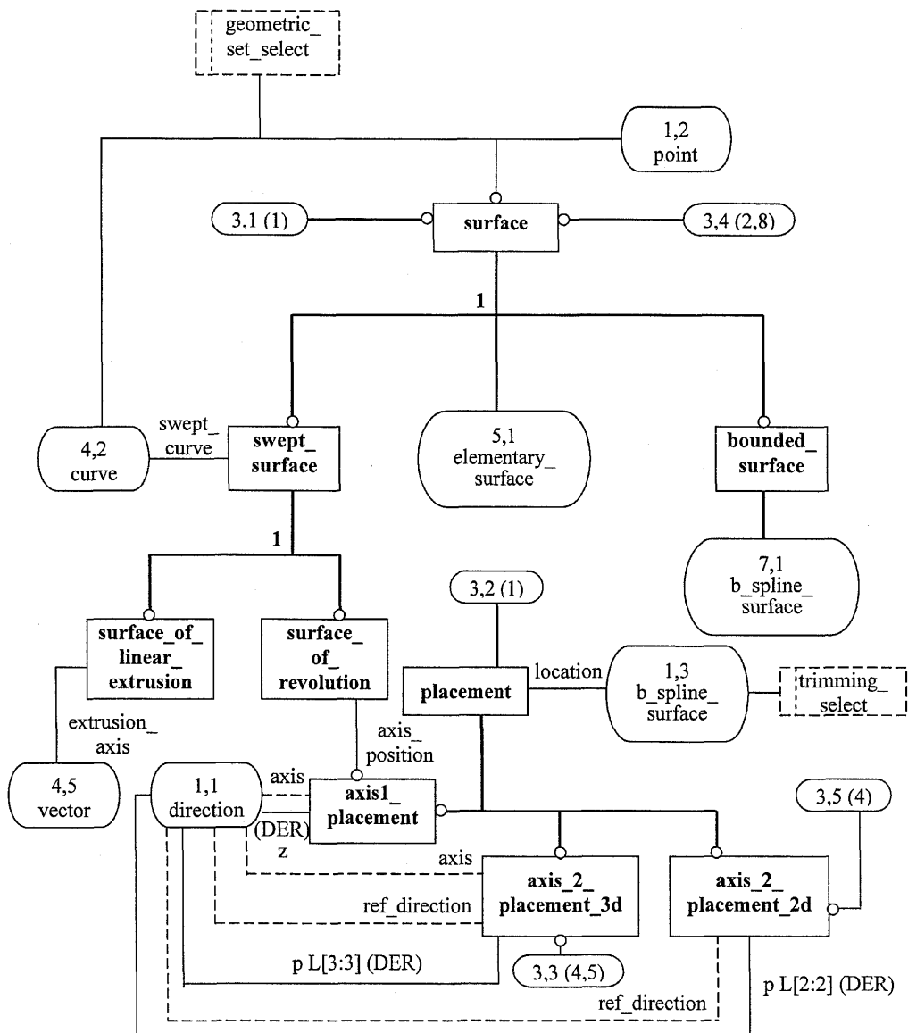
Рисунок D.3 — ПИК aic_advanced_brep в формате EXPRESS-G (диаграмма 3 из 8)
