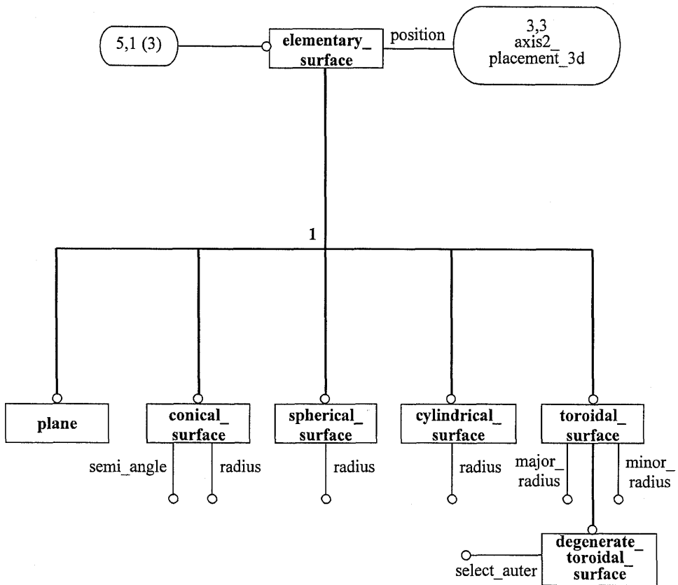
Рисунок D.5 — ПИК aic_advanced_brep в формате EXPRESS-G (диаграмма 5 из 8)
