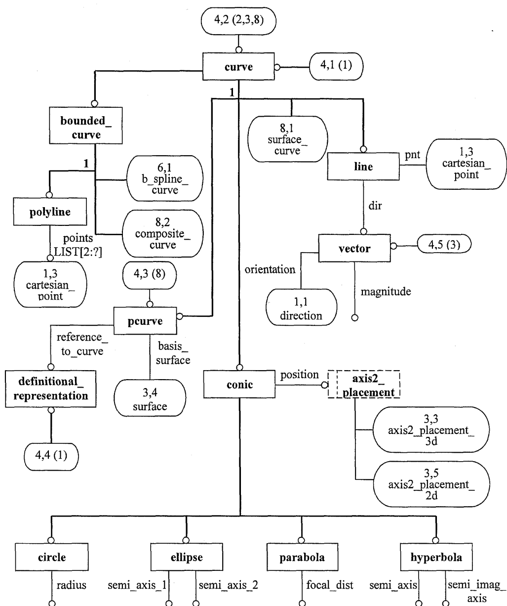
Рисунок D.4 — ПИК aic_advanced_brep в формате EXPRESS-G (диаграмма 4 из 8)
