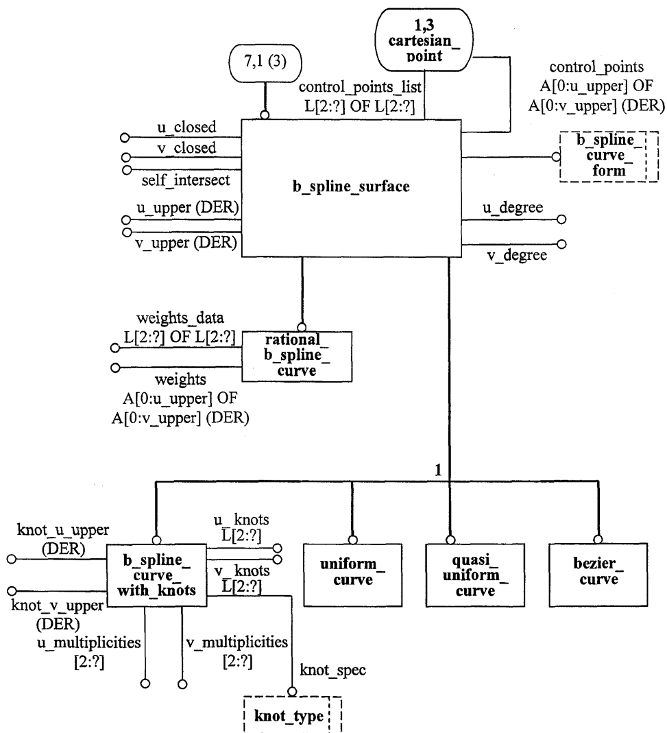
Рисунок D.7 — ПИК aic_advanced_brep в формате EXPRESS-G (диаграмма 7 из 8)
