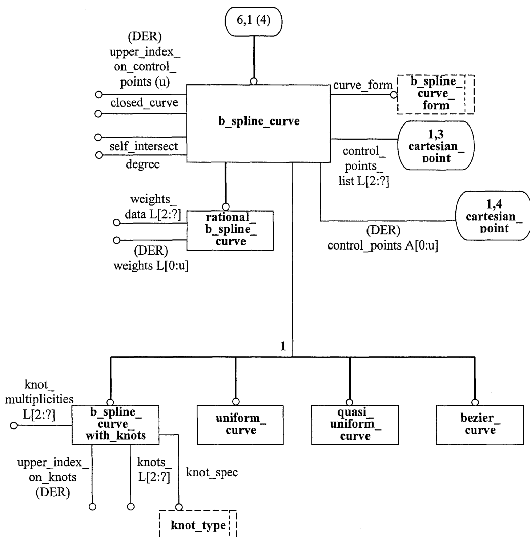
Рисунок D.6 — ПИК aic_advanced_brep в формате EXPRESS-G (диаграмма 6 из 8)
