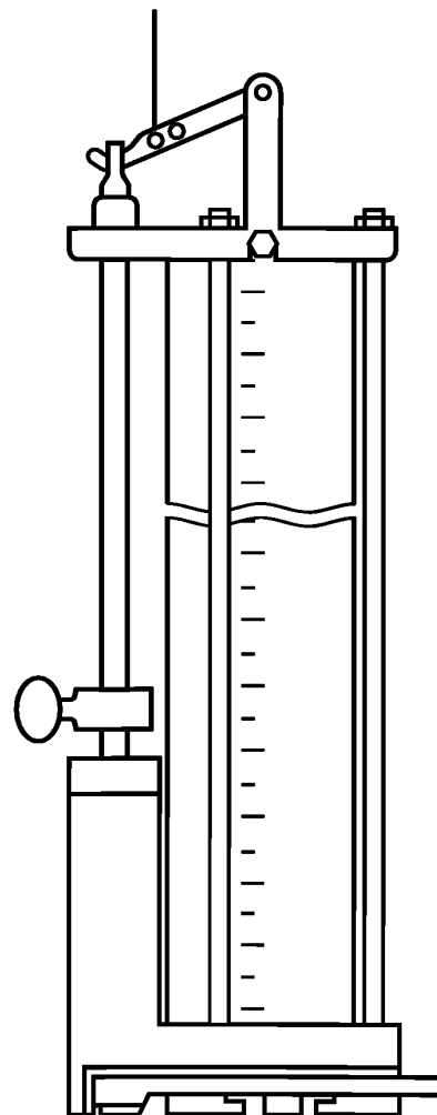
Рисунок 3 — Желонка стержневого типа для отбора проб нефтепродуктов
