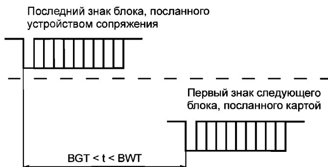
Рисунок 21 — Время ожидания блока и разграничительный интервал блока
