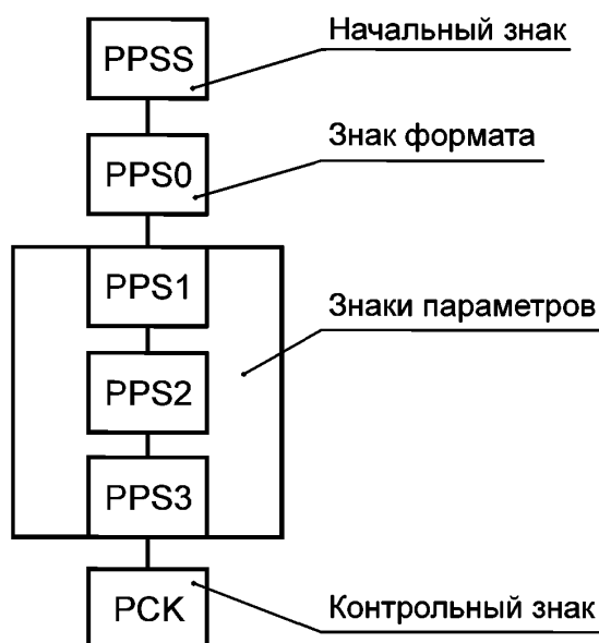
Рисунок 15 — Структура PPS-запроса и PPS-ответа
