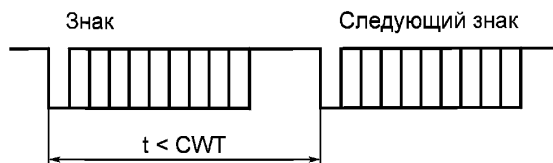
Рисунок 20 — Время ожидания знака
