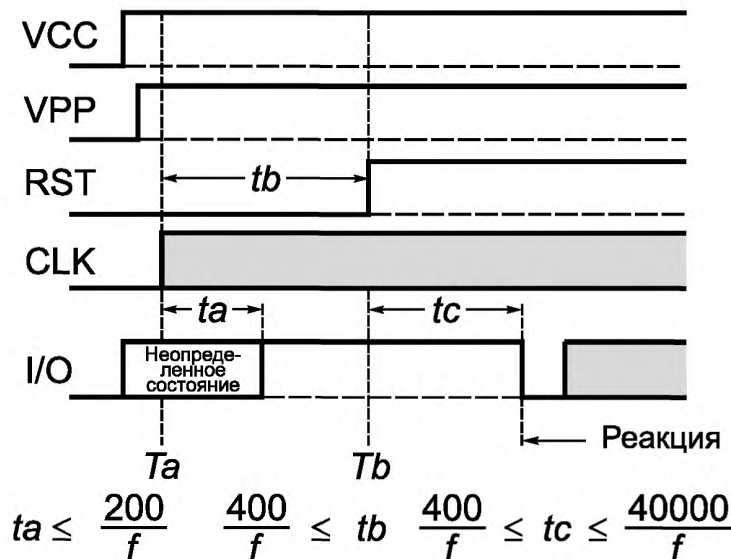
Рисунок 2 — Активизация и «холодное» восстановление
