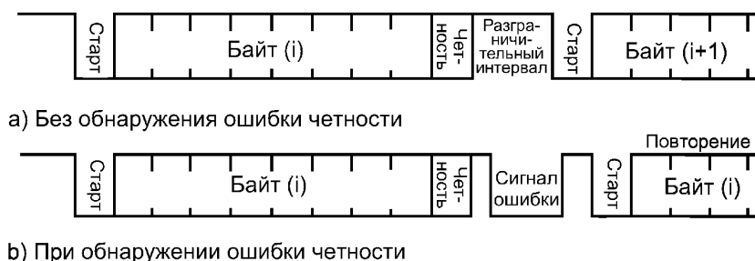
Рисунок 8 — Диаграмма передачи и повторения знака
