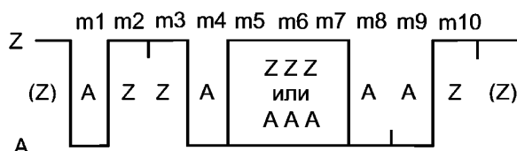
Рисунок 9 — Начальный знак TS
