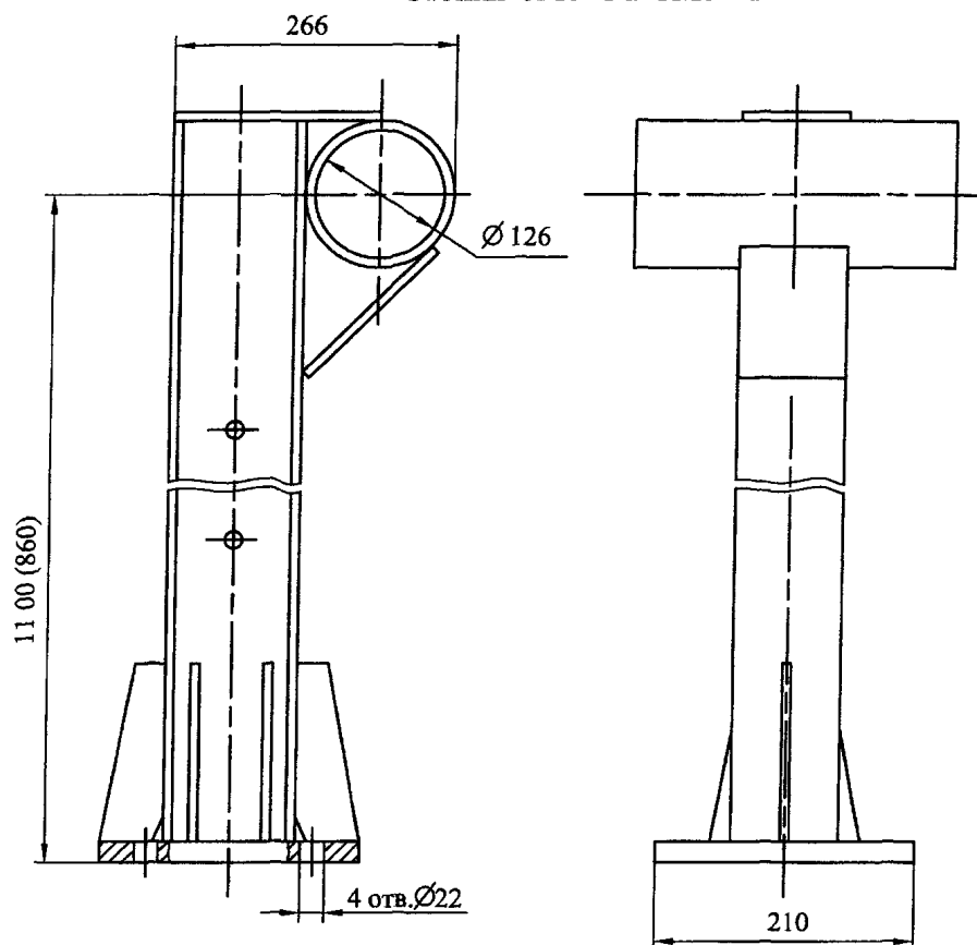
Стойки СМУ-1 и СМУ - 2
