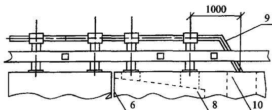
Ограждение группы 11МО-У. Концевой участок
