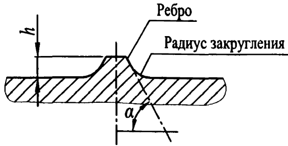
Рисунок 2 - Поперечное сечение ребра (сечение А-А из рисунка 1)
