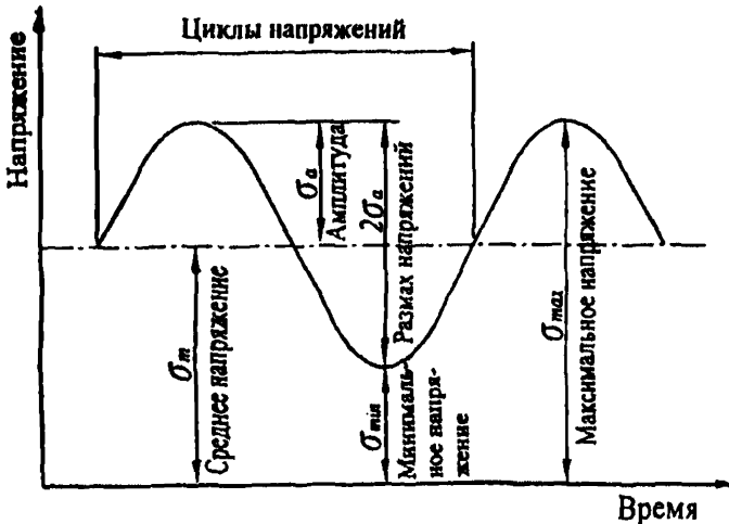
Рисунок Д.1 - Циклы напряжений при испытании на усталость
