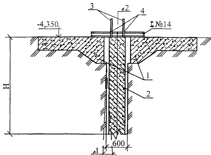
Рисунок 6 – Схема подвески панелей на стенках форшахты
