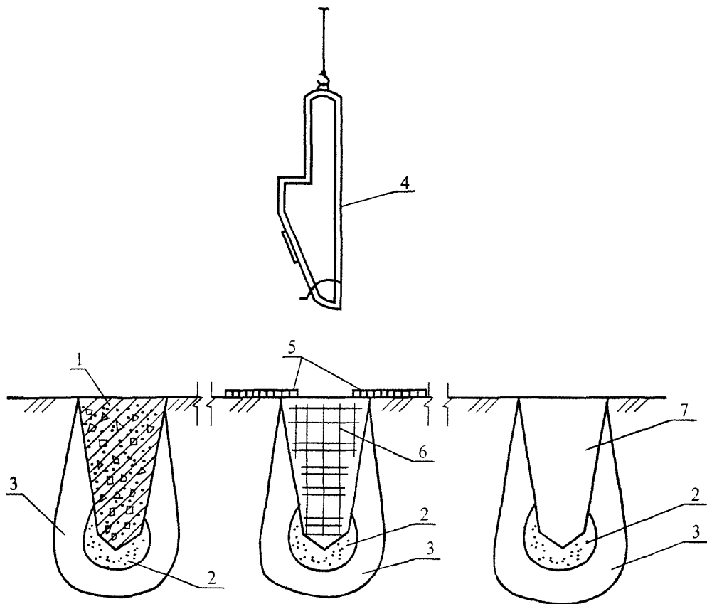
Рисунок 5 – Схема бетонирования фундаментов в вытрамбованных котлованах с уширенным основанием
