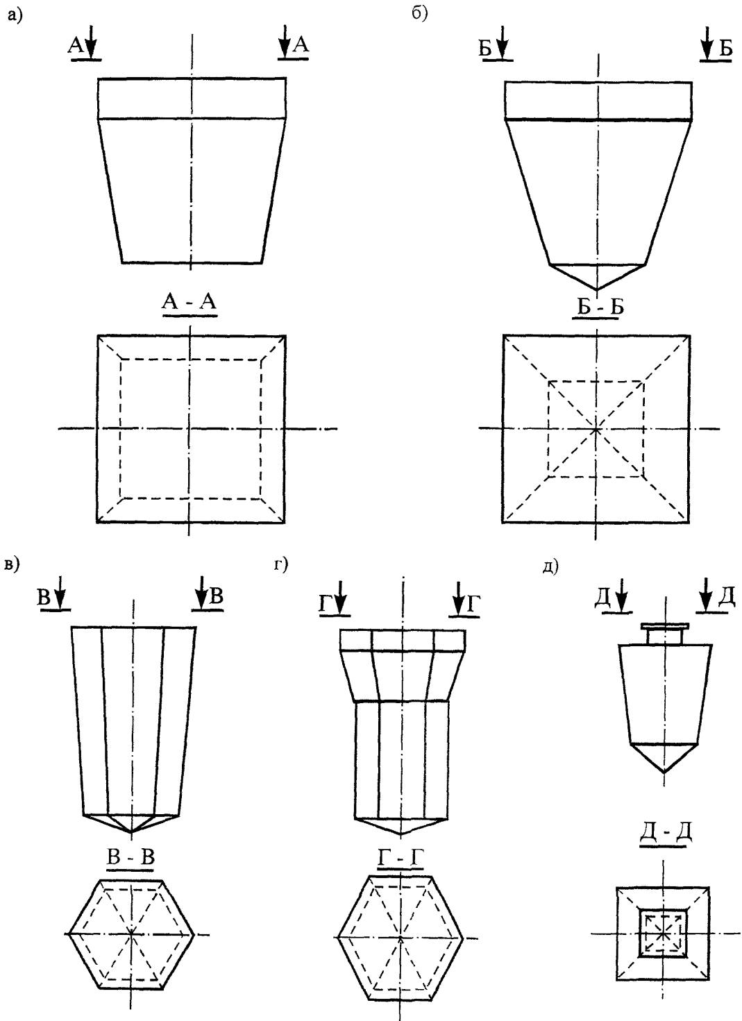
Рисунок 2 – Основные виды трамбовок для вытрамбовывания котлованов
