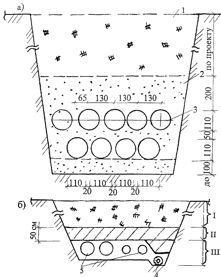
а) телефонная канализация; б) бесканальная тепловая сеть
