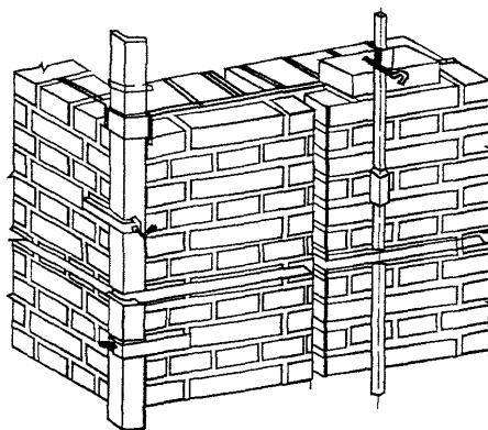
Рисунок 5 – Схема установки инвентарной металлической порядовки (шаблон)
