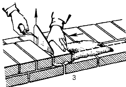
Рисунок 10 – Кладка способом «вприжим» ложкового (а) и тычкового (б) рядов наружной версты (1-3 – последовательность операций)
