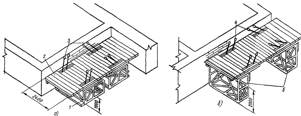
Рисунок 2 — Шарнирно-панельные подмости
