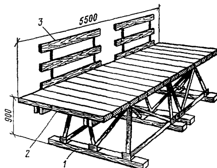
Рисунок 1 — Подмости для второго яруса кладки
