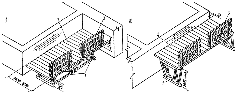
Рисунок 1 — Подмости для второго яруса кладки
