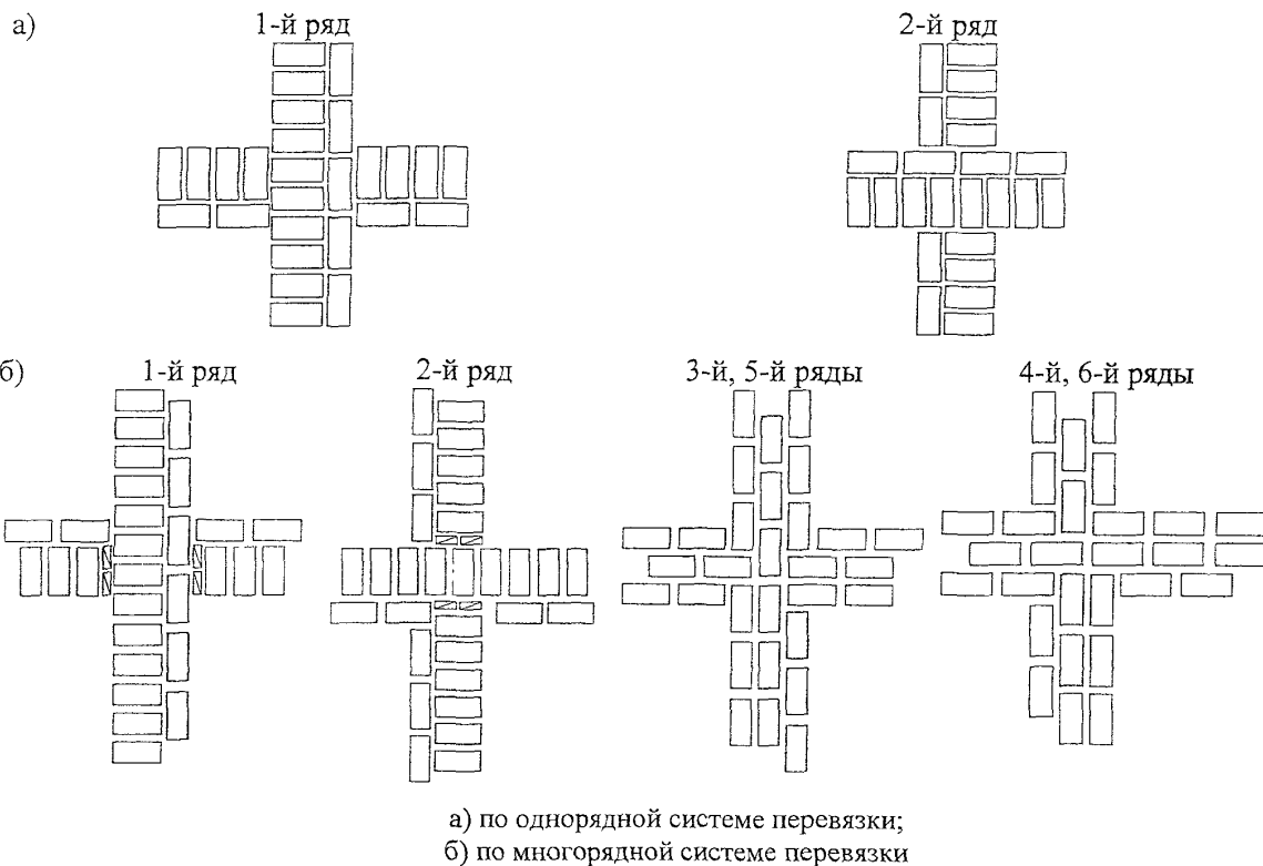
Рисунок 13 – Кладка пересечения стен толщиной в 1,5 и 1,5 кирпича
