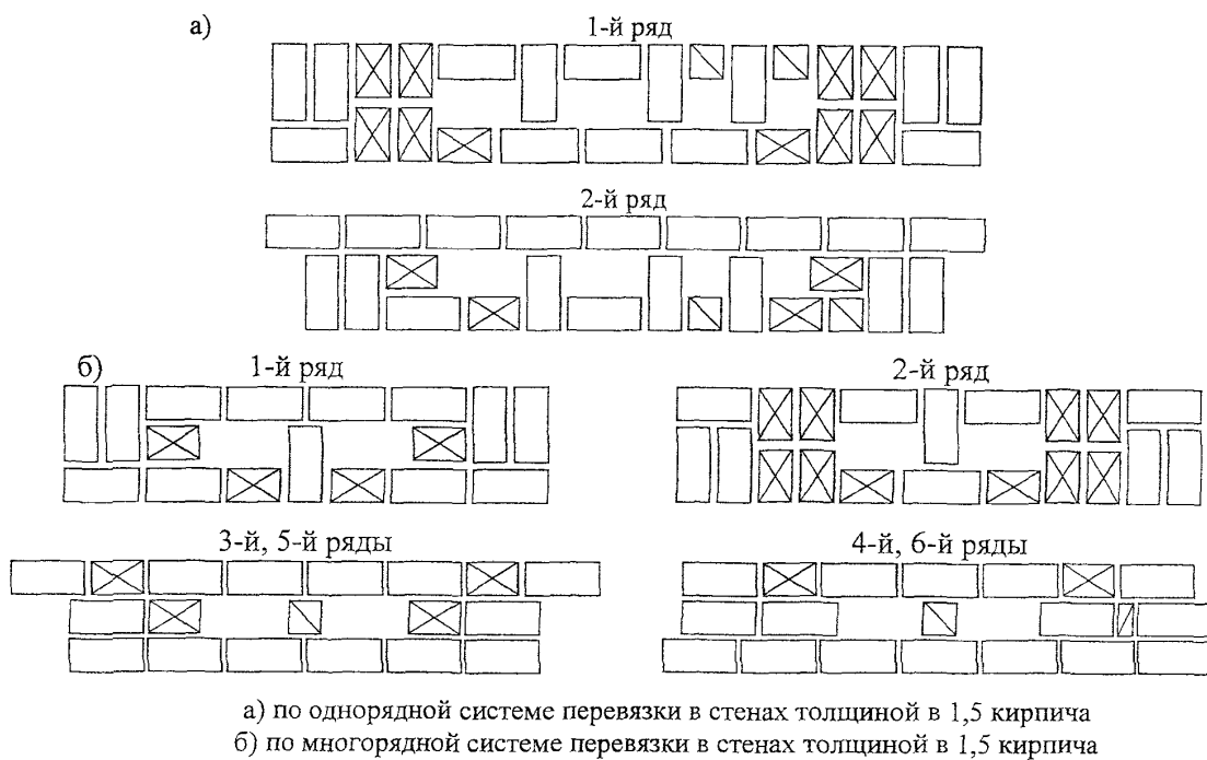
Рисунок 14 – Кладка дымовых и вентиляционных каналов
