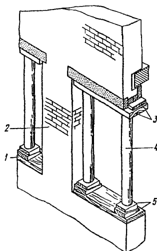
Рисунок 16 – Усиление простенков разгрузочными стойками
