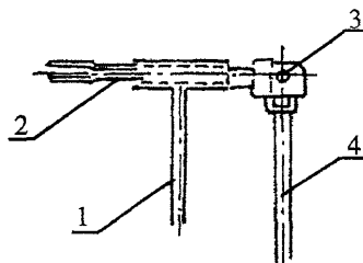
1 – вспомогательный рычаг; 2 – рабочий вал; 3 – ось; 4 – основной рычаг
