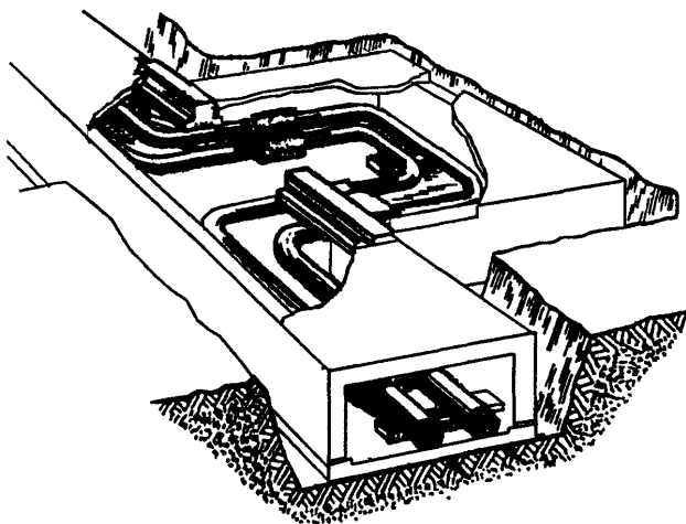
Рисунок 5 – Гнутые компенсаторы
