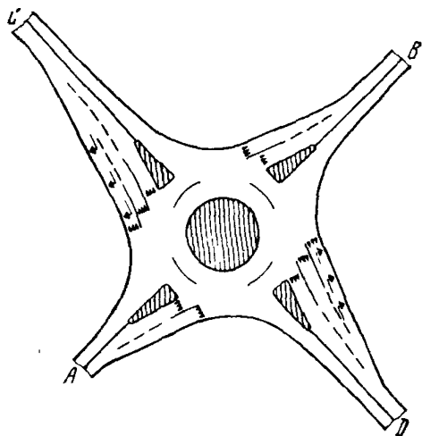
Рис. 5. Приоритет в движении на кольце
