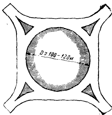
Рис 13 Кольцевое пересечение с центральным островком малого диаметра.
