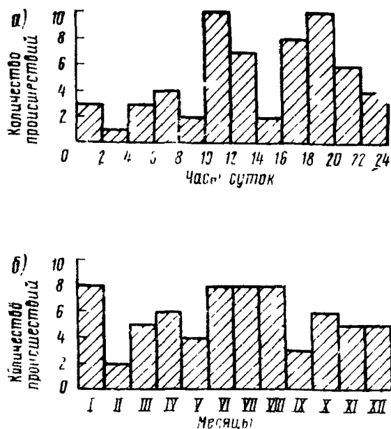
Рис 21 Распределение дорожно-транспортных происшествий на кольцевом пересечении
