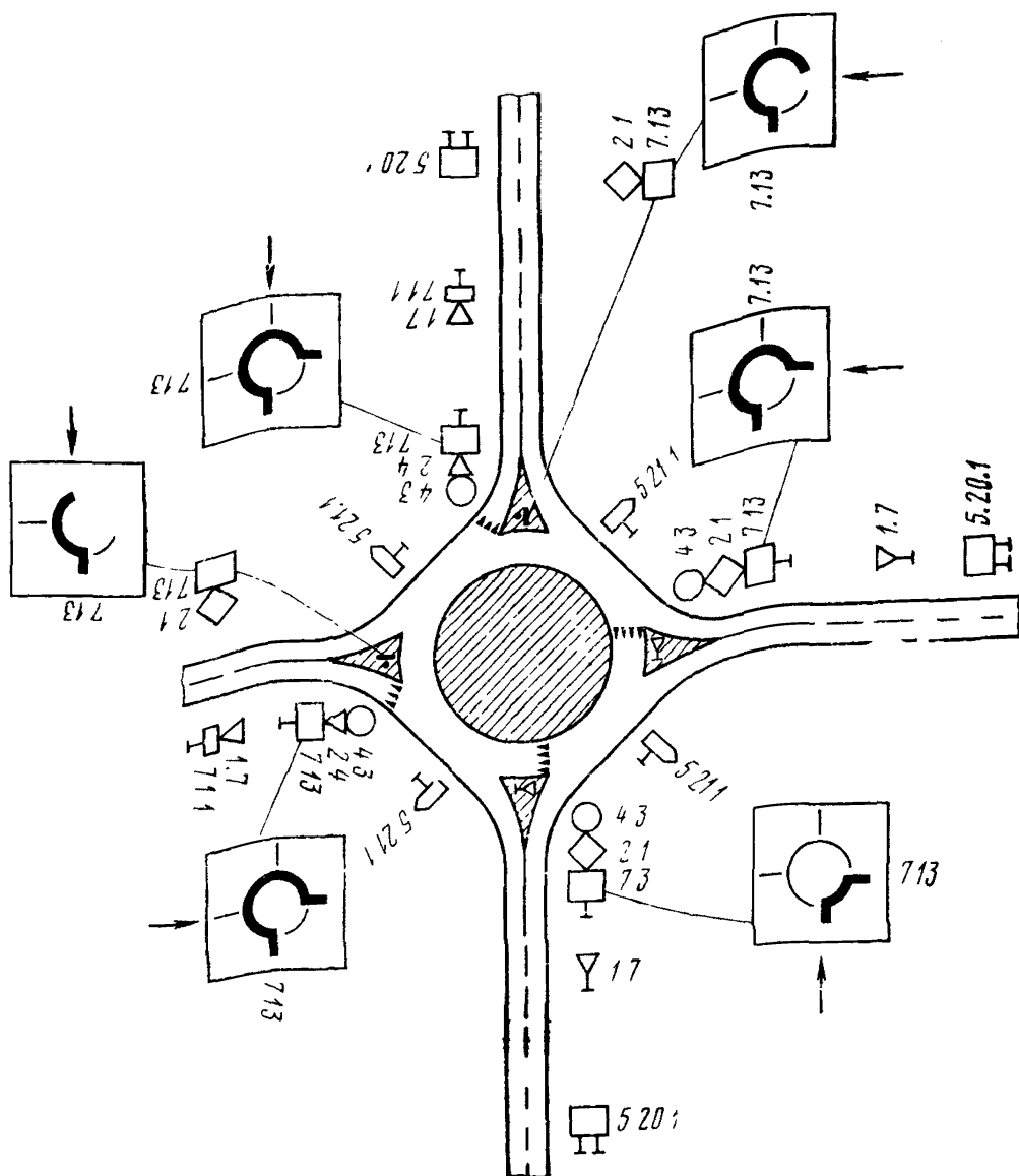
Рис 6.4. Схема расстановки знаков на кольцевых пересечениях в случае, когда главная дорога изменяет свое направление
