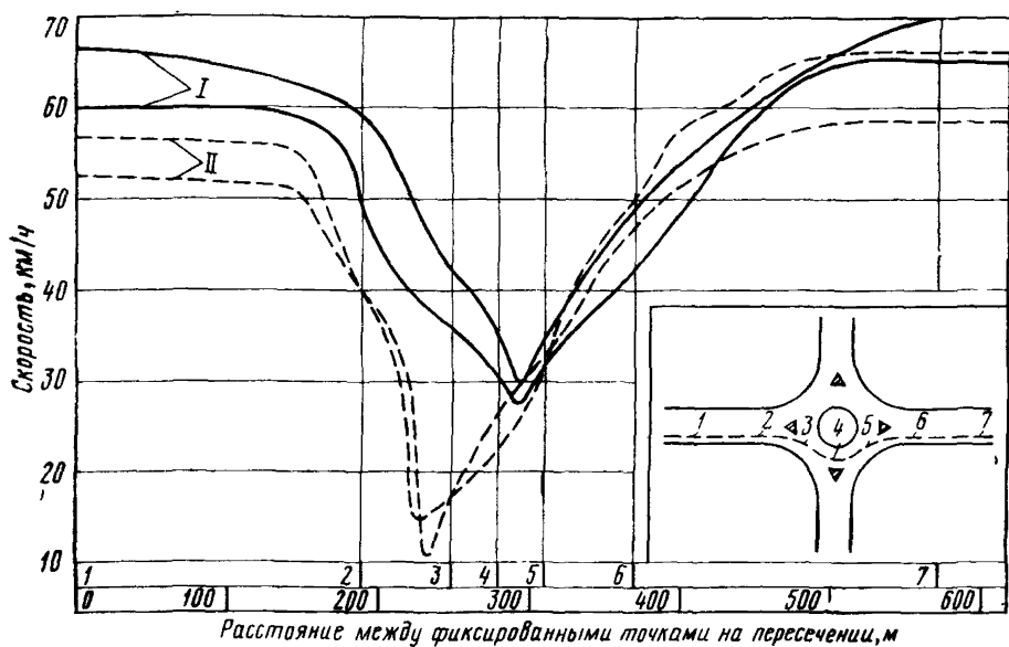
Рис 34. Изменение скорости движения на кольцевом пересечении неравнозначных дорог при проезде в прямом направлении:
