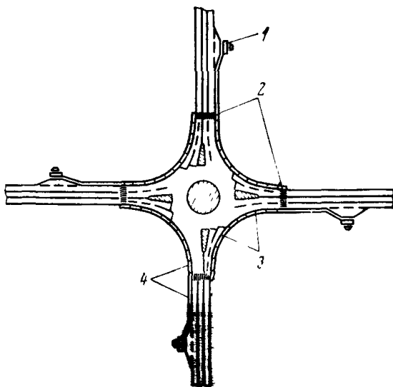
Рис 24 Схема организации пешеходного движения на кольцевом пересечении
