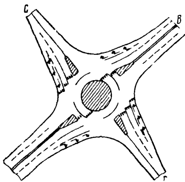
Рис 11 Направление А—В—главное
