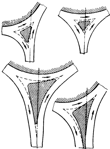
Рис 4 2 Виды направляющих островков кольцевых пересечений автомобильных дорог
