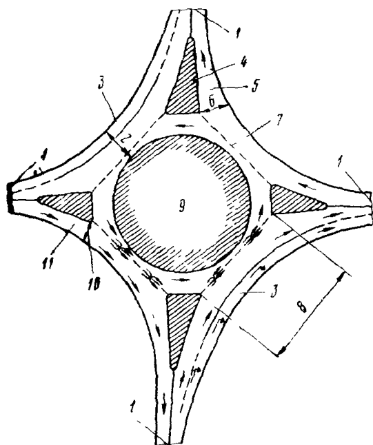
Рис 11. Элементы кольцевого пересечения
