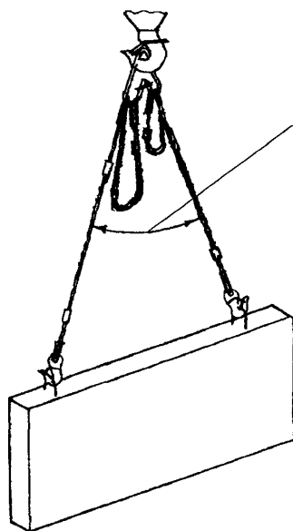
Строп 4СК1-3,2; 4СК1-5,0; 4СК1-10,0; (2СК-5,0); Q = 5,0 \div 10,0 тс Q = 3,2 \div 10,0 тс, Q = 5,0 \div 10,0 тс при монтаже стеновых панелей P = 0,71 \div 2,45 т
