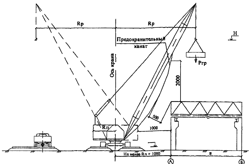
Рис. 10. Вертикальная привязка стреловых кранов с предохранительным канатом:
