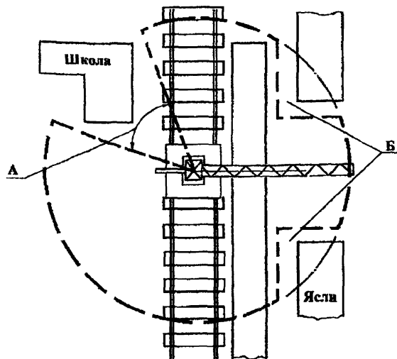
Рис. 26. Схема действия системы ограничения зон работы (СОЗР) башенного крана:
