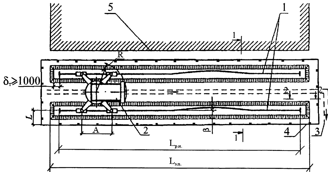
Рис. 39. Общий вид и основные контролируемые параметры наземных рельсовых крановых путей на деревянных полушпалах (начало):
