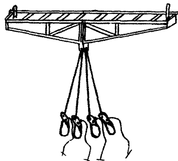
Траверса для подъема ферм покрытия двумя кранами
