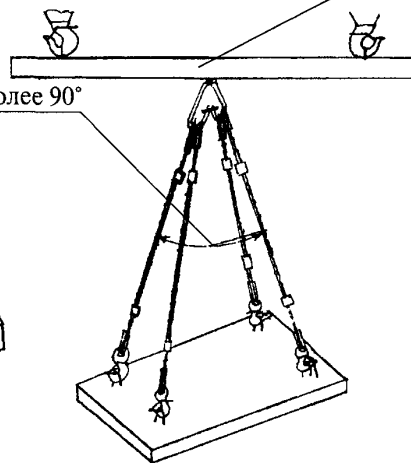
Строп 4СК1-5,0 + 4СК1-10,0 Q = 5,0 \div 10,0 тс при монтаже двумя кранами
