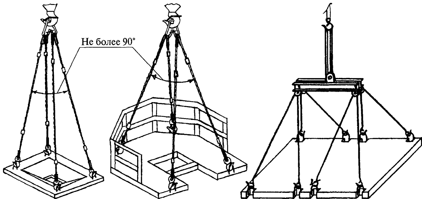
Строп 4СК1-3,2÷4СК1-10,0 Q = 3,2 \div 10,0 тс при монтаже капитальных плит
