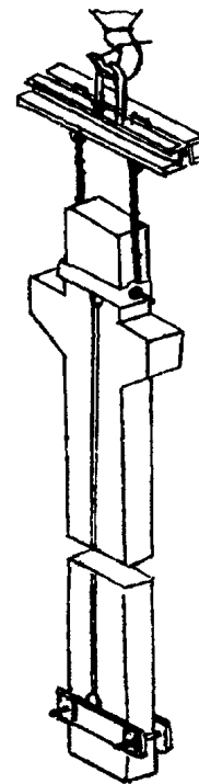
Универсальный захват Q = 6,0 тс для монтажа колонн массой до 6,0 \text{ т}
