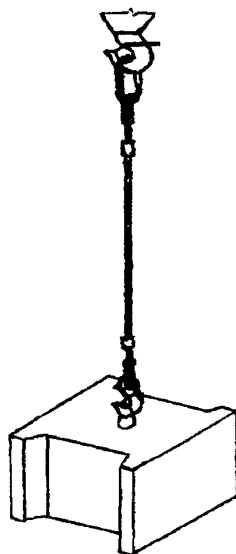
Строп одноветевой Q = 2,5 тс при монтаже блоков стен подвала P = 0,98 \div 1,97 т
