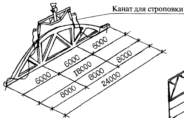
Траверса ТР20-5,0 L = 5,0 \text{ м} , Q = 20 \text{ тс} для монтажа железобетонных ферм P до 16 т
