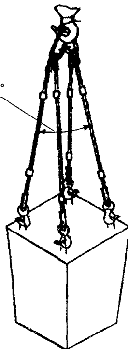
Строп 4СК1-3,2÷4СК1-10,0 Q = 3,2 \div 10,0 тс при разгрузке с транспорта подколонников P = 2,5 т
