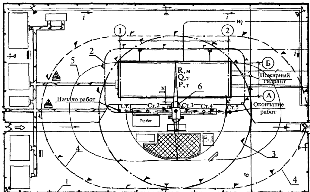
Рис. 13. Границы зон при работе стрелового крана (крана-манипулятора):
