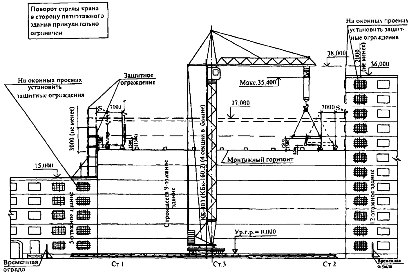
Рис. 22. Разрез 1-1
