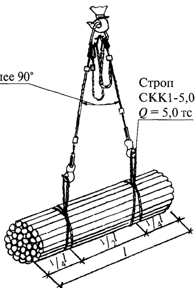
Строп 4СК1-3,2+4СК1-10,0 Q = 3,2+10,0 тс при подаче арматурных стержней P = 1,0 т
