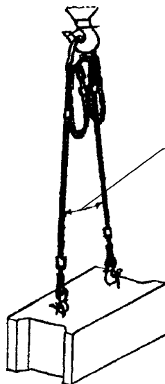
Строп 2СК-3,2÷2СК-10,0 Q = 3,2 \div 10 тс при монтаже блоков стен подвала P = 0,31 \div 0,62 т
