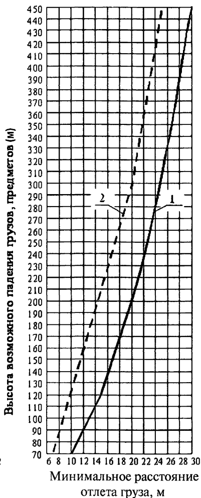
Рис. 15. График определения минимального расстояния отлета груза при его падении:
