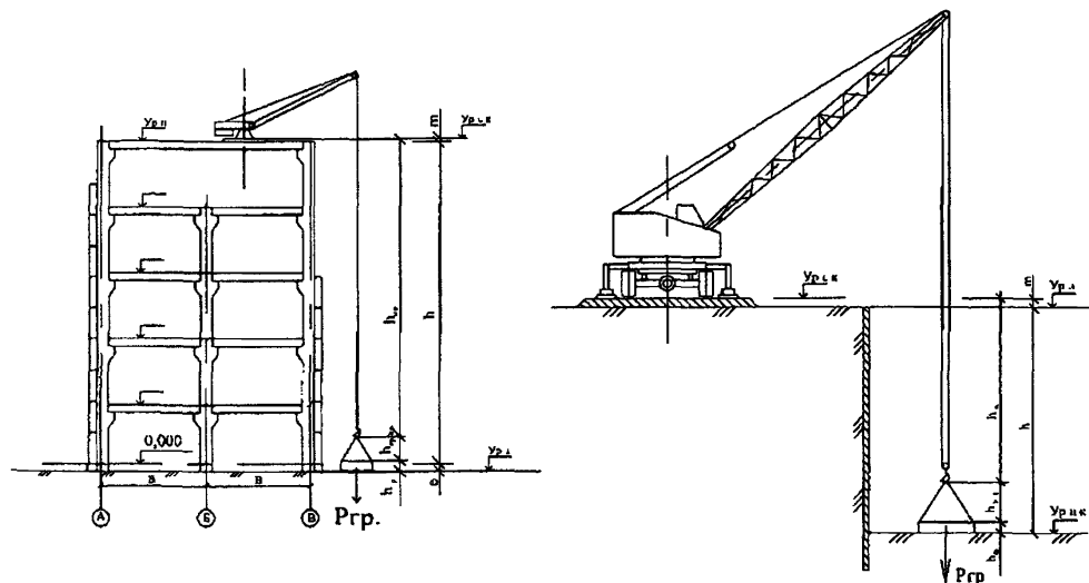
Рис. 4. Установка кранов для опускания (подъема) грузов ниже уровня стоянки:
