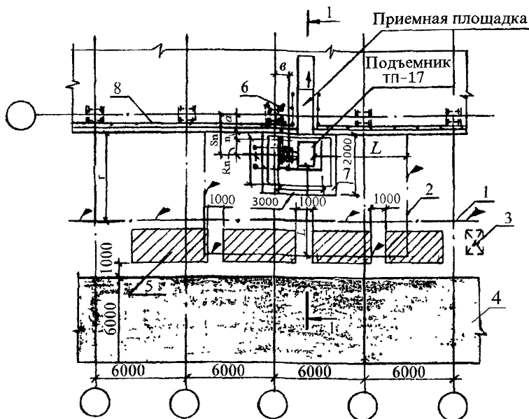
Рис. 37. Подача грузов на крышу здания с помощью подъемника ТП-17 (начало):
