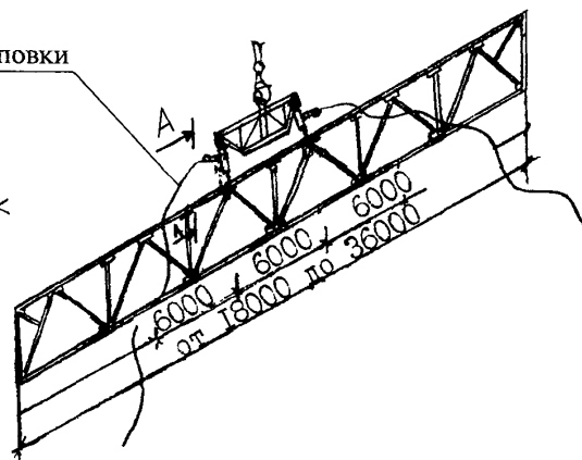
Траверса ТР20-5,0 L = 5,42 \text{ м} , Q = 20 \text{ тс} для монтажа металлических ферм P = 3,9 \div 15 \text{ т}
