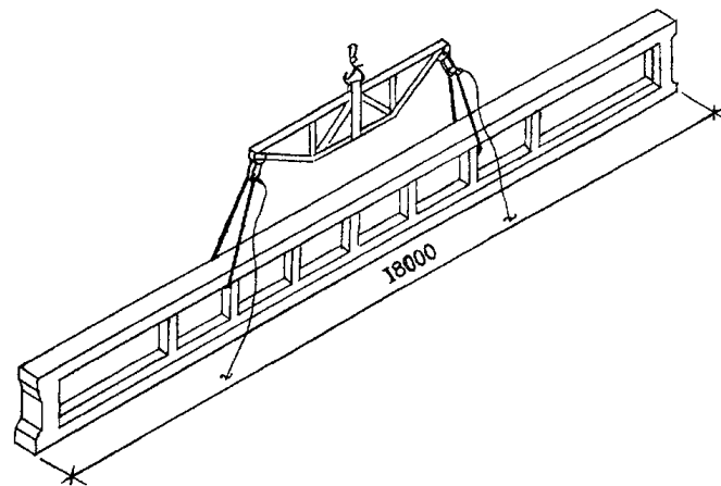
Траверса ТР20-5
