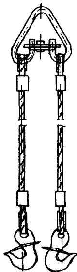
Строп канатный двухветвевой типа 2СК ГОСТ 25573–82*
