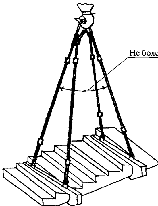
Грузозахватное приспособление Q = 2,1 тс для монтажа лестничных маршей массой до 2 т
