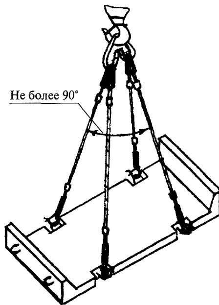
Строп 4СК1-3,2÷10,0 Q = 3,2 \div 10,0 тс при погрузке лоткового днища канала P = 0,74 \div 2,85 т
