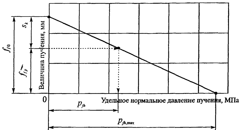
Рисунок 3.1 К определению величины удельного давления морозного пучения p_{\text{ж}} путем расчета по формуле (2.8) с учетом допустимого (возможного) перемещения фундамента на величину f_{\text{жр}}
