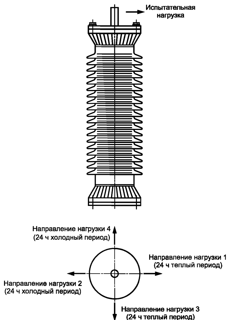
Рисунок 5 — Направления действия изгибающей нагрузки при термомеханических испытаниях
