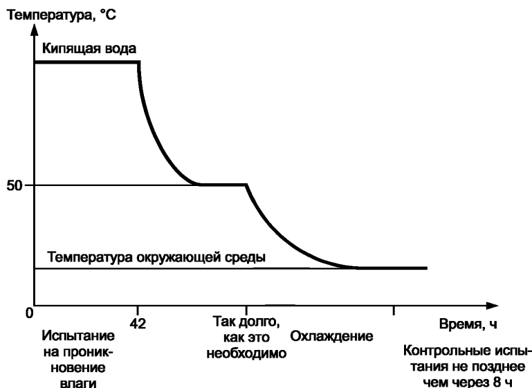
Рисунок 6 — Испытания на проникновение влаги
