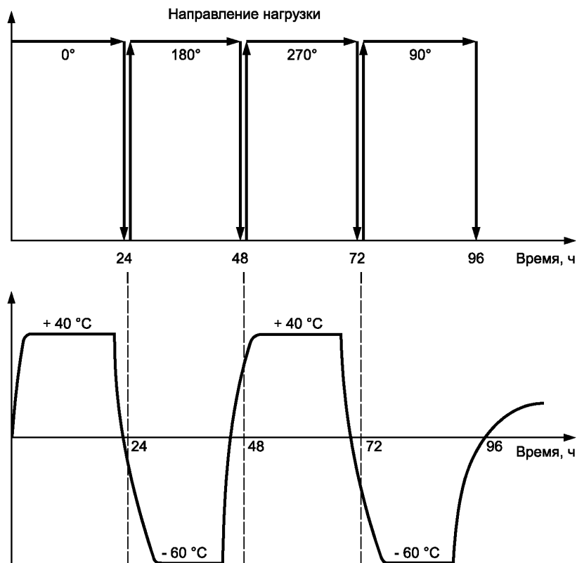
Рисунок 4 — Термомеханические испытания
