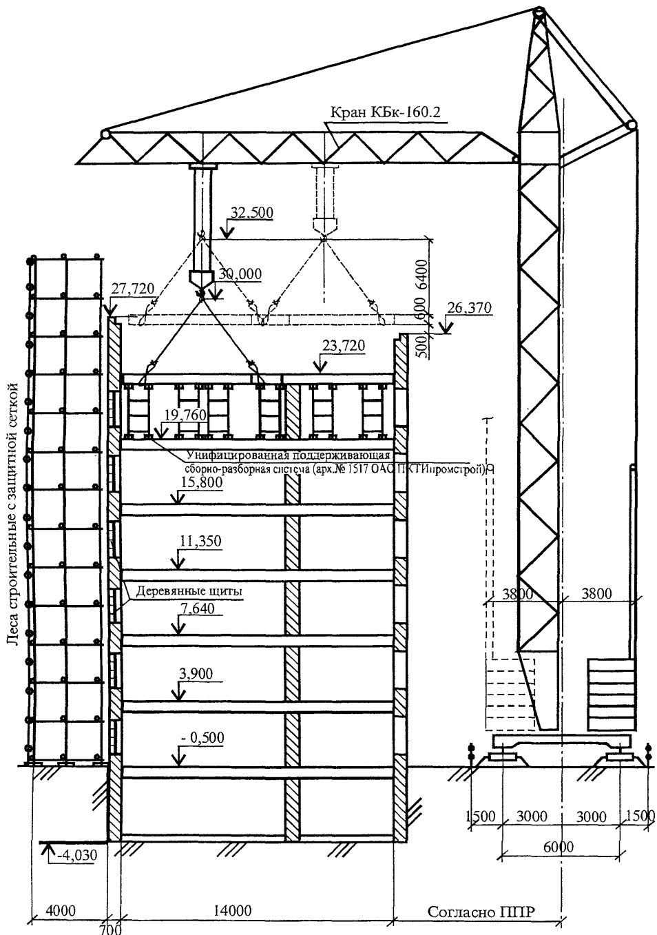
Рисунок 7 – Схема привязки крана на период разборки перекрытий
