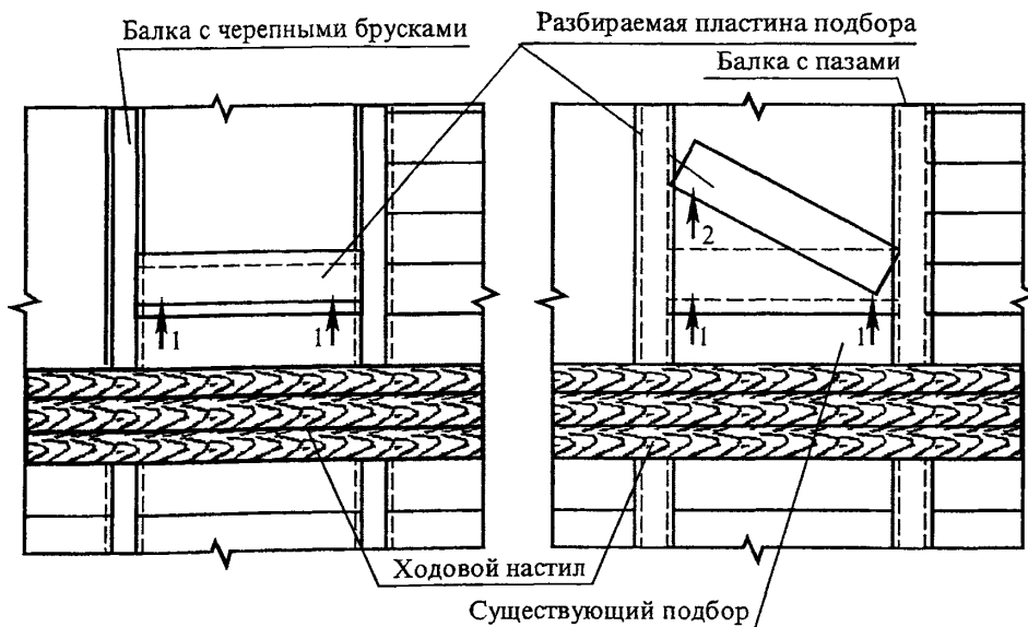
Рисунок 6 – Схема разборки деревянного подбора
