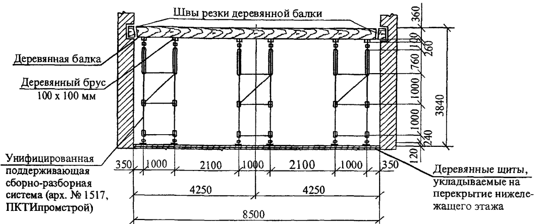
Рисунок 8 – Схема разборки междуэтажного перекрытия по деревянным балкам
