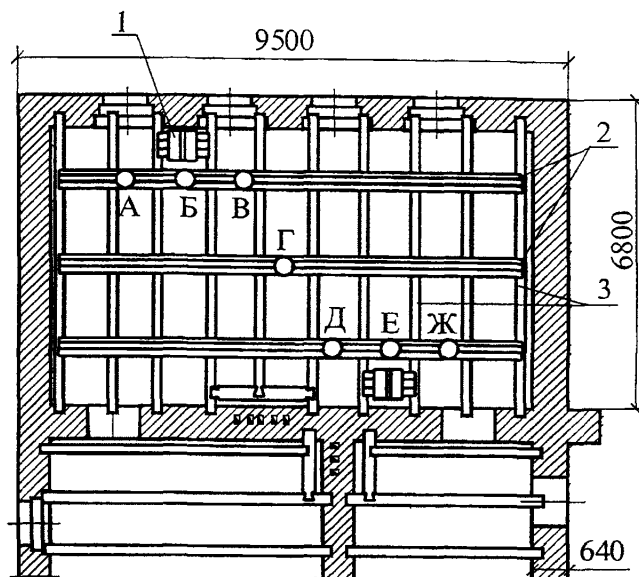
Рисунок 9 – Схема организации работ на захватке
