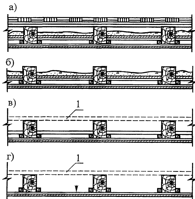
Рисунок 2 – Последовательность разборки элементов междуэтажного перекрытия с паркетным полом
