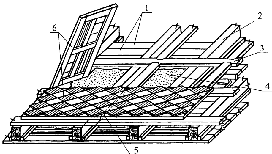
Рисунок 4 – Разборка щитового паркетного пола
