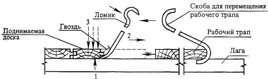
Рисунок 3 – Схема разборки чистых полов из шпунтованных досок и брусьев
