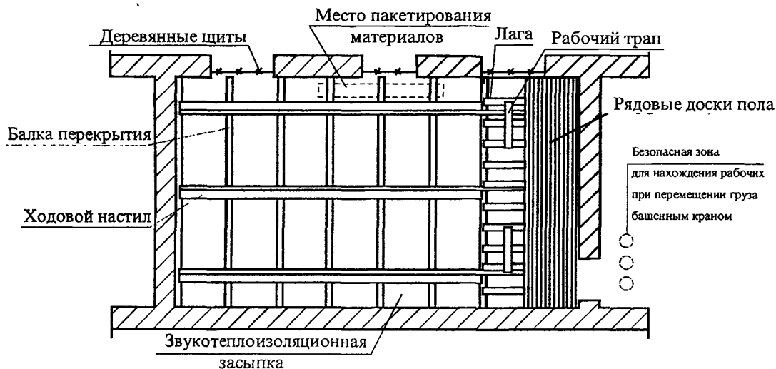
Деталь разборки
