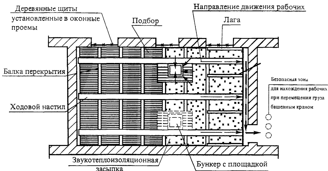
Рисунок 5 – Схема удаления звукотеплоизоляции (засыпки) перекрытия
