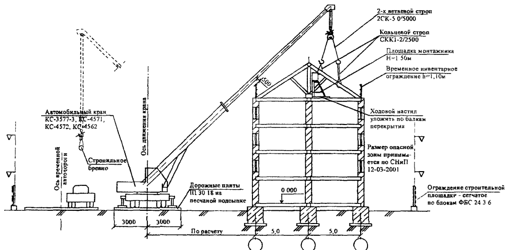
Рисунок 5 – Схема строповки стропильных балок
