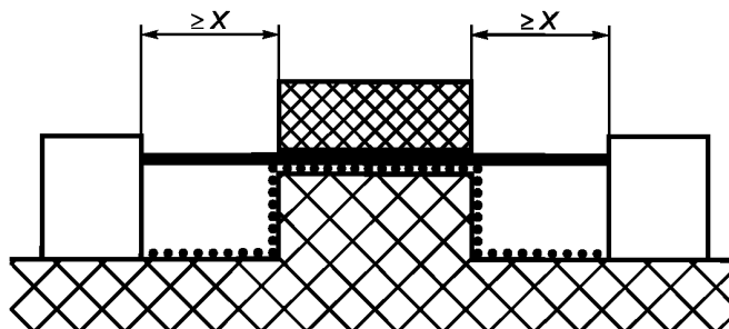
Рисунок E.6 — Несплошной стык с широкими канавками
