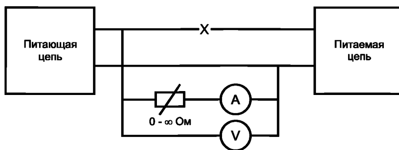
Рисунок 1 — Схема испытательной цепи для условий неисправности
