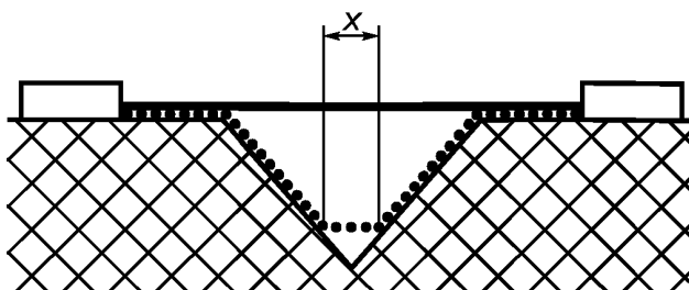
Рисунок E.3 — V-образная канавка
