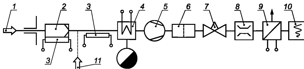
1 — зонд для отбора пробы; 2 — фильтр для удаления твердых частиц; 3 — нагревательная оболочка; 4 — охладитель пробы с сепаратором конденсата; 5 — насос для прокачивания пробы; 6 — фильтр; 7 — вентиль тонкой регулировки; 8 — расходомер; 9 — газоанализатор; 10 — регистратор данных; 11 — отверстие для ввода калибровочной газовой смеси, содержащей диоксид серы, и нулевого газа
