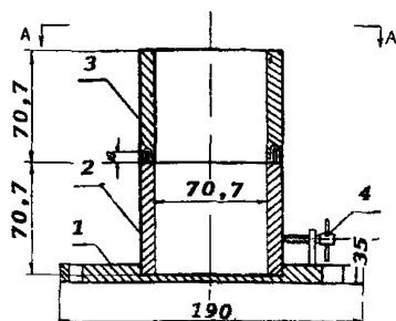
б. форма для изготовления образцов из литой смеси II и III типов
