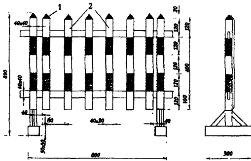
Пакетный барьер облегченного типа
