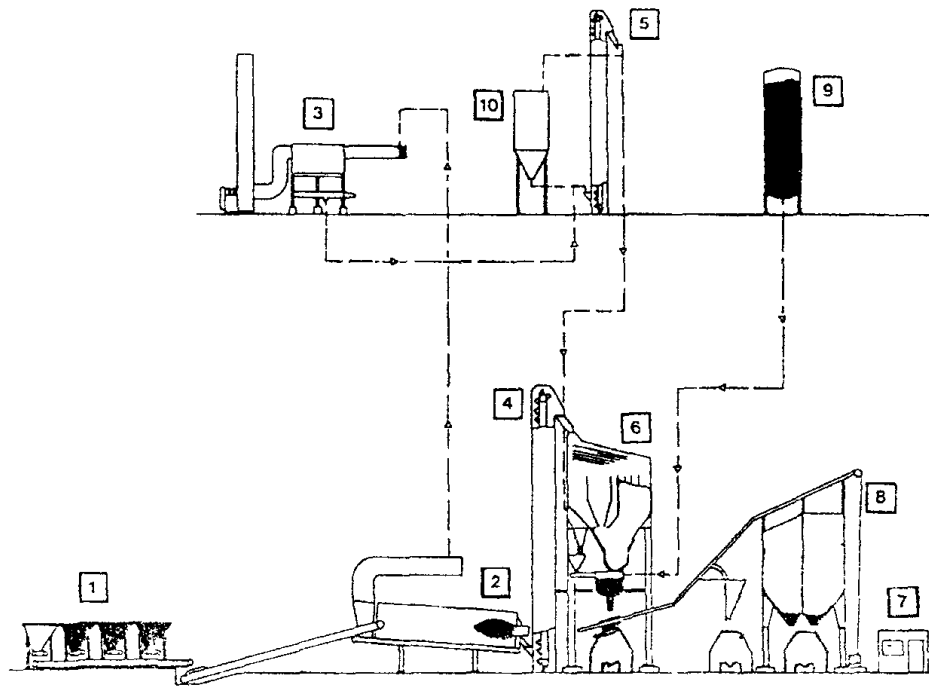
Рис.1. Схема технологического процесса приготовления ливной асфальтобетонной смеси
