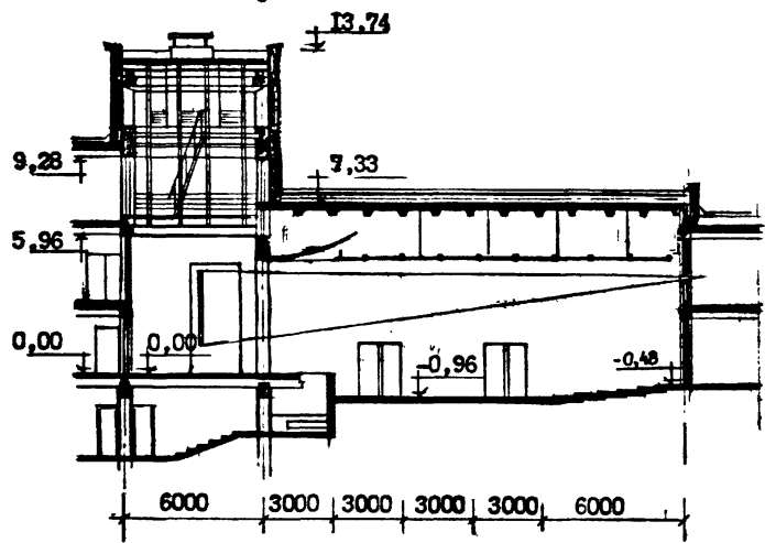
Разрез А-А
