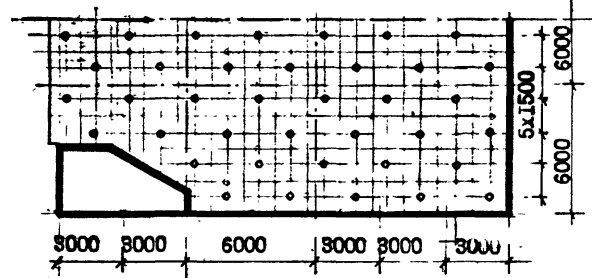
План разбивки светильников подвесного потолка
