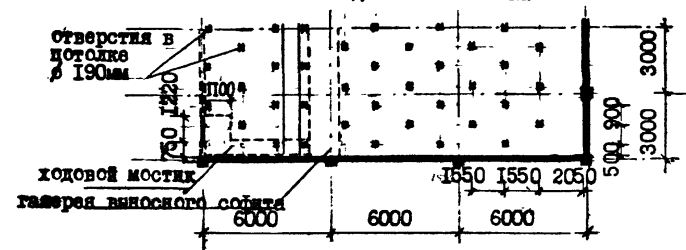
План разбивки светильников подвесного потолка
