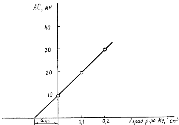
Рисунок 4 - Зависимость аналитического сигнала от объема введенных в электролизер градуировочных растворов \text{Cu(III)} , \text{Pb(II)} и \text{Cd(II)}
