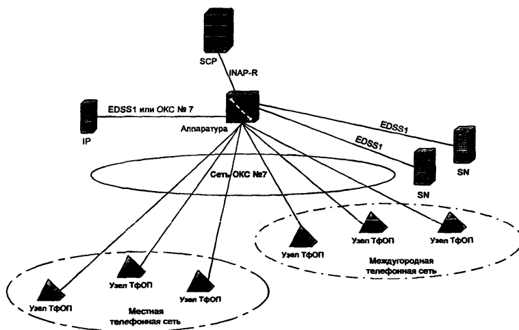
Рисунок 4.1 – Взаимодействие аппаратуры с узлами телефонной сети общего пользования и узлами платформы ИСС
