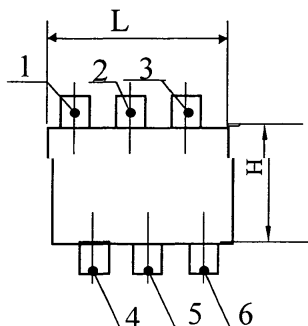
Коробка КСП-63-10, КС-25-20, КС-25-30, КСП-25-20, КСП-25-25
