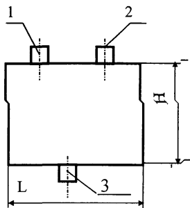
Коробка КС-25-10, КС-63-10
