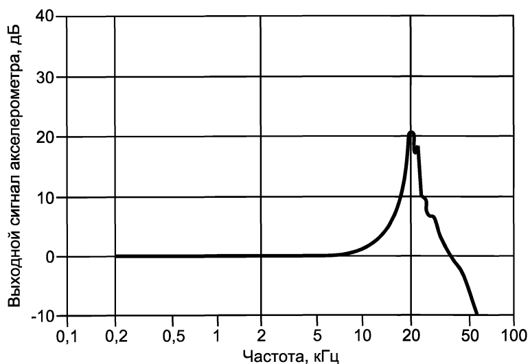
Рисунок 9 — Частичная частотная характеристика акселерометра на магните
