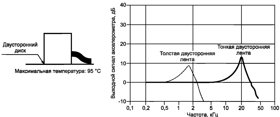
Рисунок 7— Типичная частотная характеристика акселерометра, установленного с помощью ленты с двусторонней клеевой поверхностью
