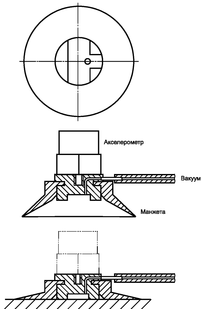
Рисунок 11 — Вакуумное крепление
