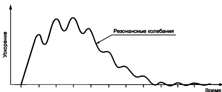
Рисунок 4 — Отклик акселерометра на удар
