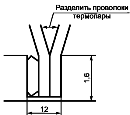
b) укрепление провода в термопаре.
