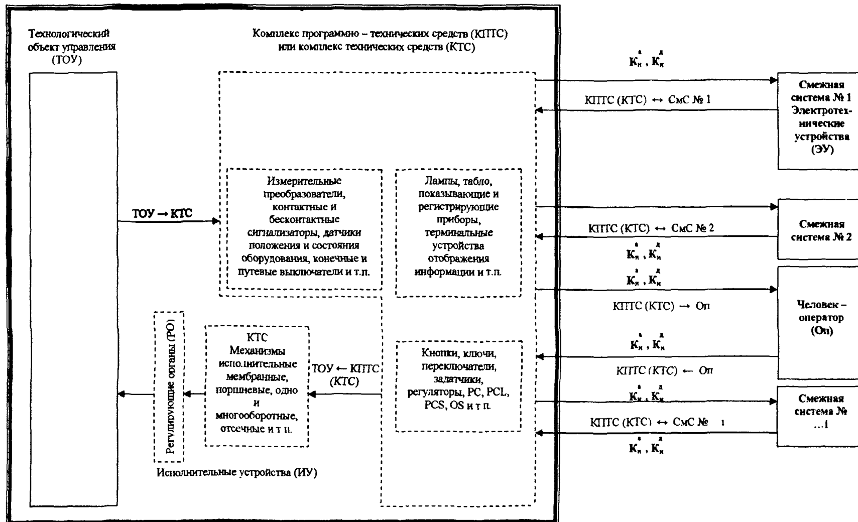
Схема автоматизированного технологического комплекса (АТК)
