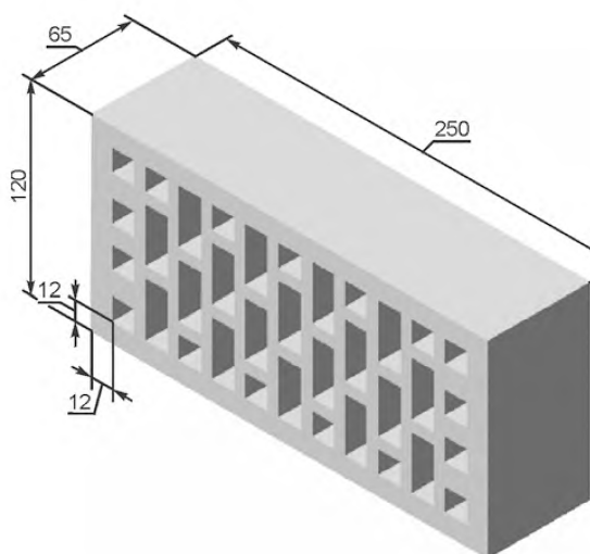
Рисунок А.1.9 — Кирпич формата 1 НФ с 35 пустотами
