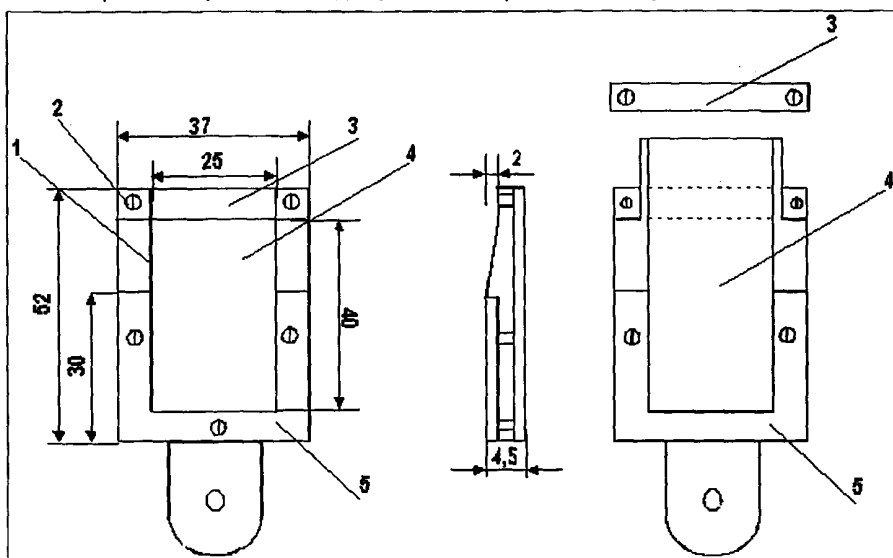
Рис.Ж.1. Общий вид диффузионного прибора.
