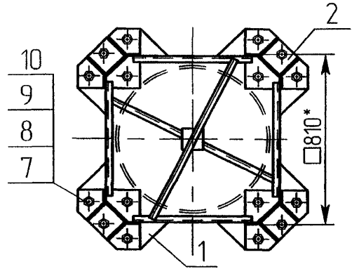
Вид Г подвеска натяжная изолирующая (поз. 22) условно не показаны М1·20
