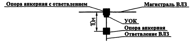
Схема №2 - для концевой опоры
