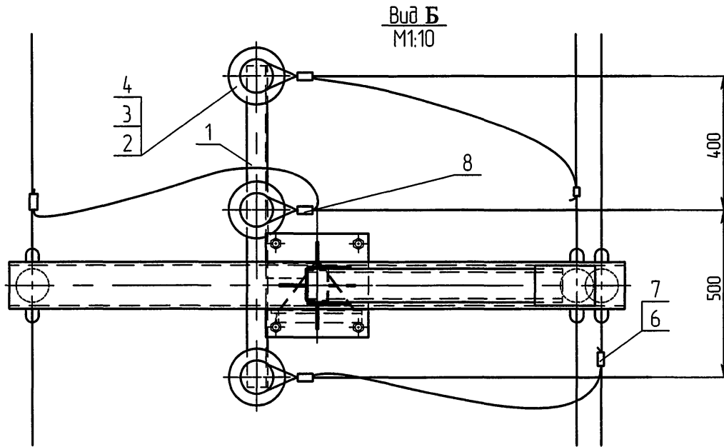
Схема установки опоры на ВЛЗ
