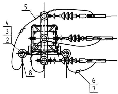
Вид В M1:10
