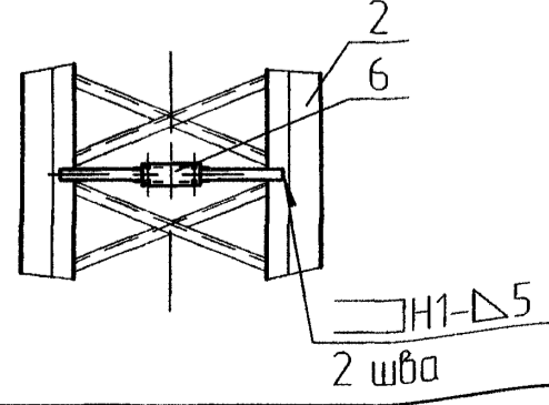
Вид Ж привод (поз 22) условно не показан М1:20
