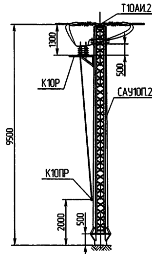
ЭЛ-ТП.010.06-31
