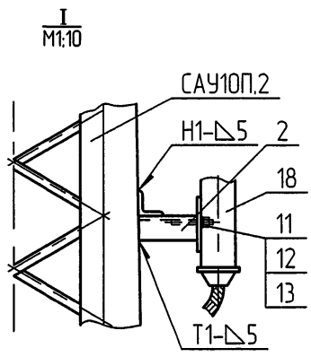
Схема установки опоры на ВЛЗ
