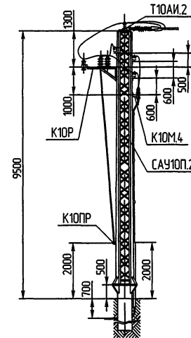
ЭЛ-ТП.010.06-35
