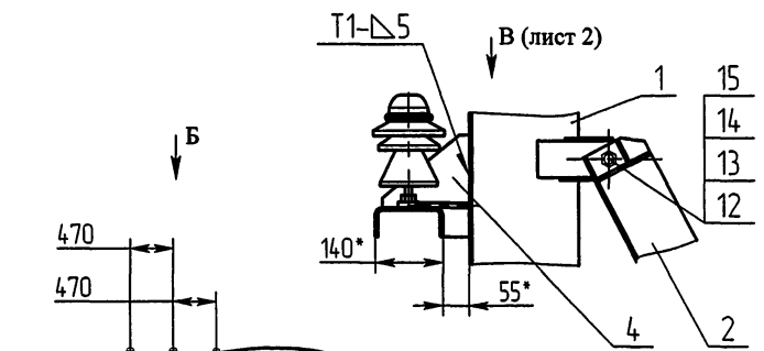
I M1:10 подвеска натяжная изолирующая (поз. 29) условно не показана
