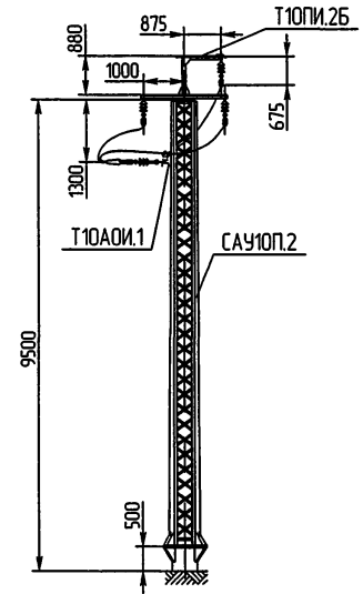
ЭЛ-ТП.010.06-19
