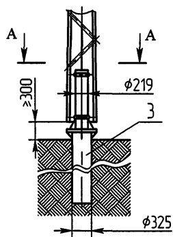
Вариант установки опоры на фундамент ФС10.219/325
