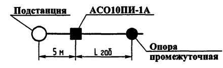
Схема №2 - для концевой опоры
