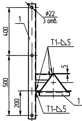
А-А поз. 2, 3 и 4 условно не показаны М1:10
