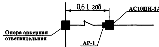
установка опоры с разъединителем на ответвлении ВЛЗ
