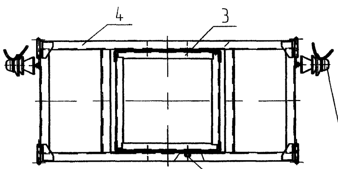
В-В подвеска натяжная изолирующая (поз 26) M1 20 условно не показаны
