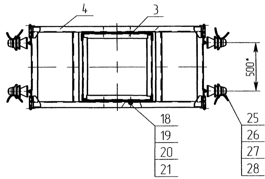
В-В подвеска натяжная изолирующая (поз 24) условно не показаны М1:20
