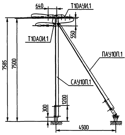
ЭЛ-ТП.010.06-20
