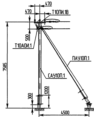
ЭЛ-ТП.010.06-16
