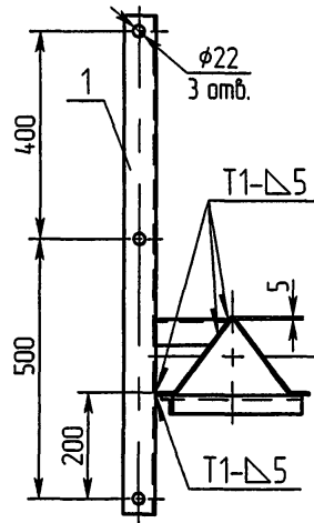
A-A поз. 2, 3 и 4 условно не показаны M1:10
