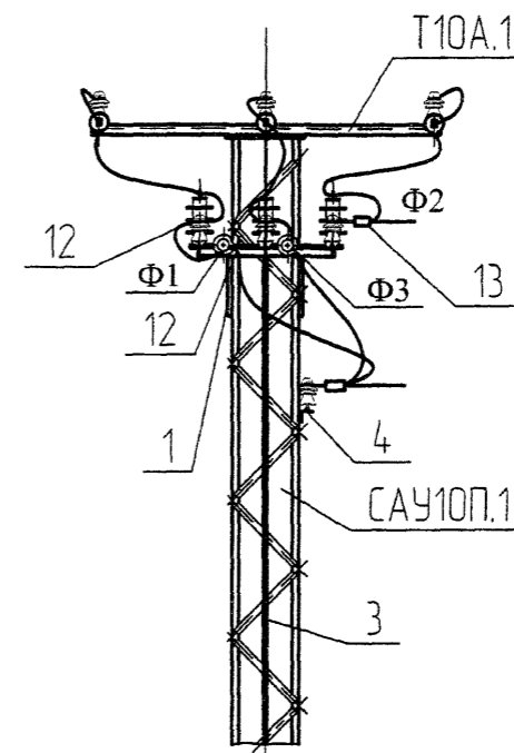
Вид Б (лист 1)
