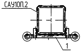
A-A M1:20 поз. 2, 3 и 4 показаны условно
