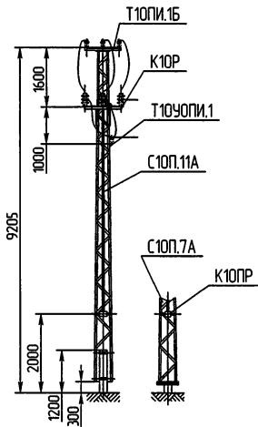
ЭЛ-ТП.010.06-26
