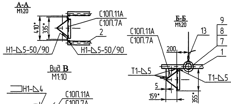
Схема установки опоры на ВЛЗ
