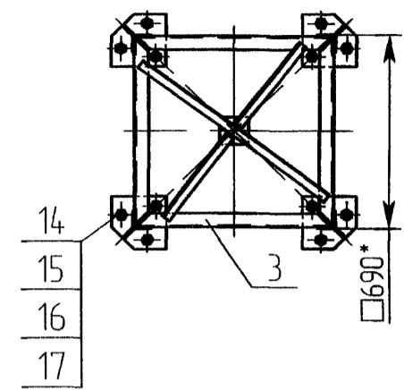
Вид Г подвеска натяжная изолирующая (поз 24) условно не показаны М1:20
