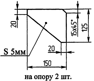
Поз. 4 Косынка материал 09Г2С
