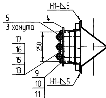
Д-Д (вариант II) М1:10
