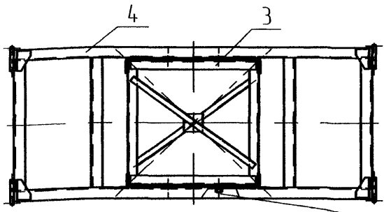
Вид Г подвеска натяжная изолирующая (поз 22) условно не показаны
