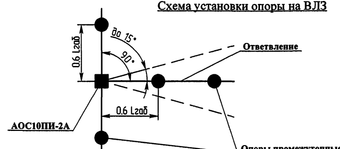
III (лист 2) Схема установки опоры на ВЛЗ
