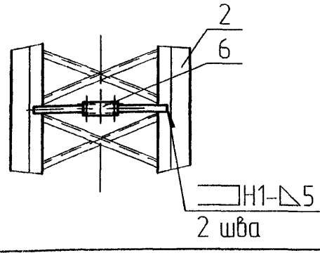
Вид Ж привод (поз 22) условно не показан M1.20
