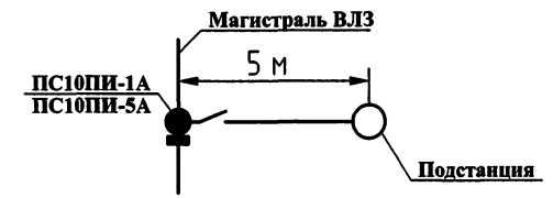
Схема установки опоры на ВЛЗ
