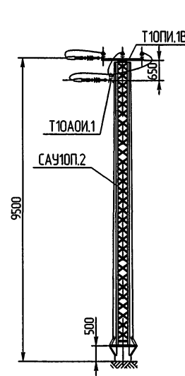
ЭЛ-ТП.010.06-18
