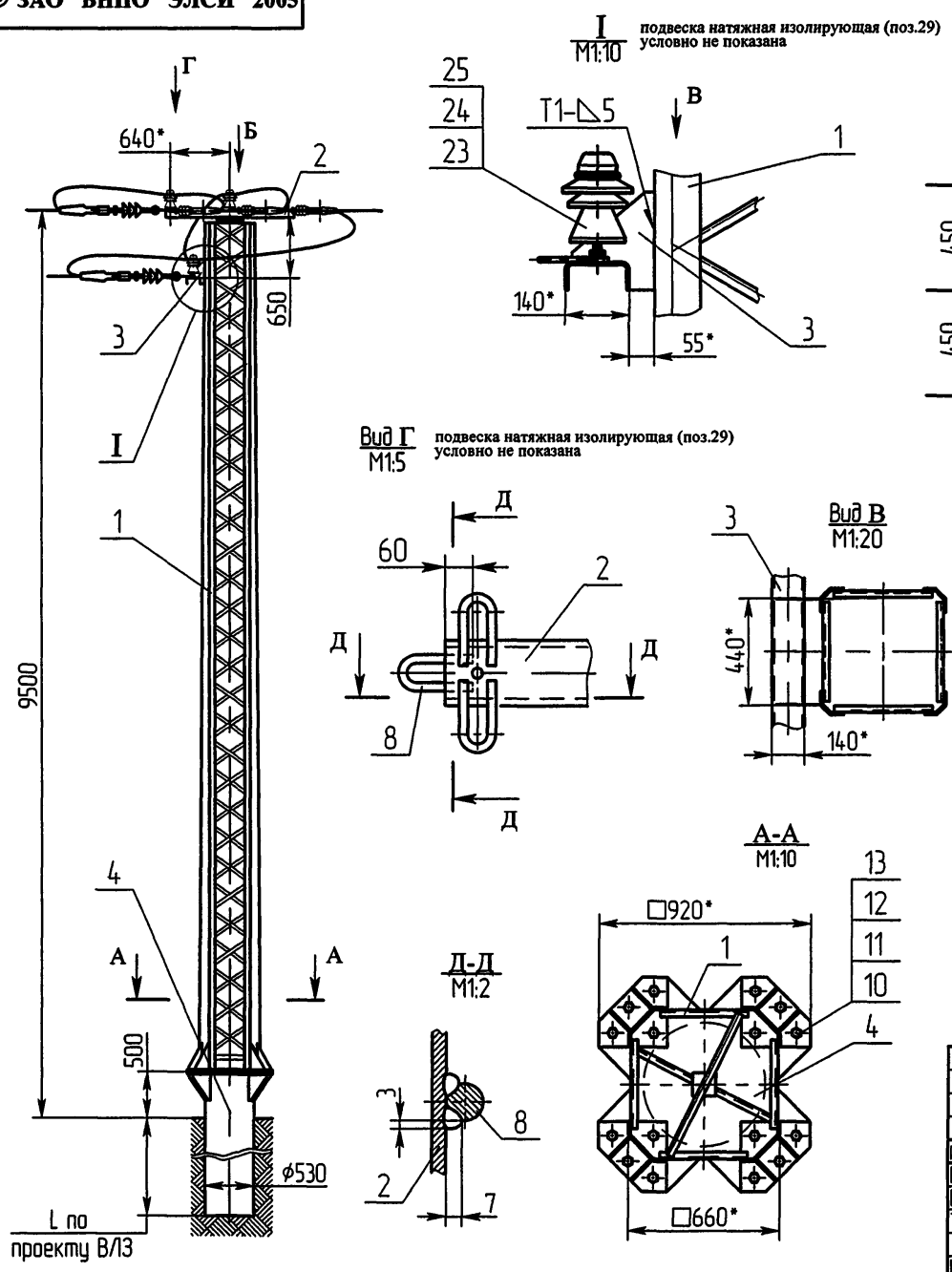
Схема установки опоры на ВЛЗ
