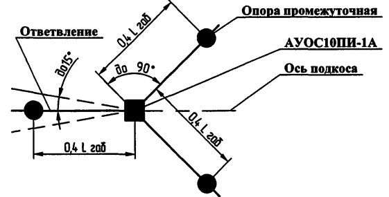
Схема установки опоры на ВЛЗ
