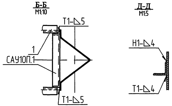
Схема установки опоры на ВЛТ
