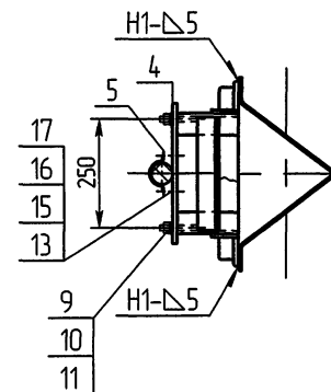
Д-Д (вариант I) М1:10
