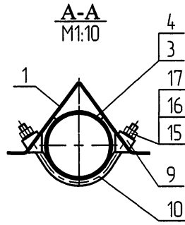
Вариант установки опоры на фундамент ФС10.219/325
