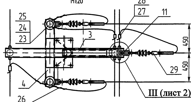
III (лист 2) Схема установки опоры на ВЛЗ
