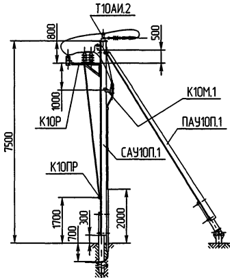
ЭЛ-ТП.010.06-34
