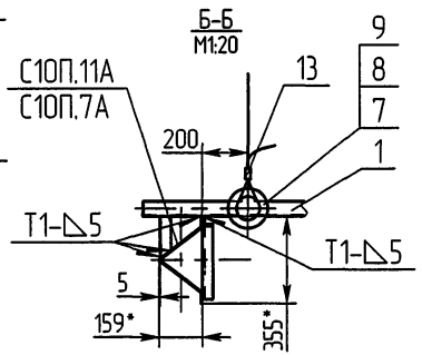
Схема установки опоры на ВЛЗ
