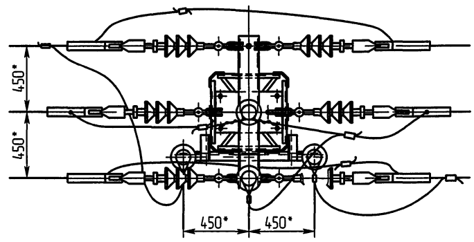
Вид Б (Схема для анкерной опоры) M1:20
