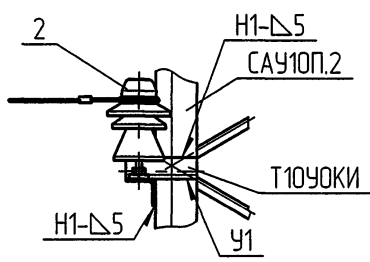
Вид В M1:10
