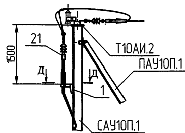
Д-Д (вариант II) М1:10
