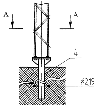
Вариант установки опоры на фундамент \Phi 10.219
