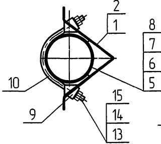
A-A M1:10
