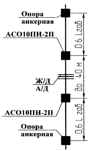
Схема установки опоры на ВЛЗ
