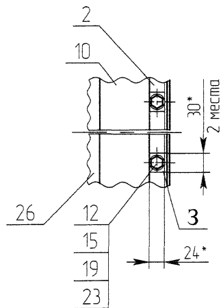
Вид Е M15
