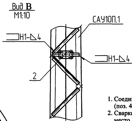
установка опоры с разъединителем на ответвлении ВЛЗ
