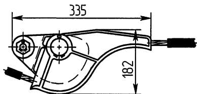
НЗ-2-7
