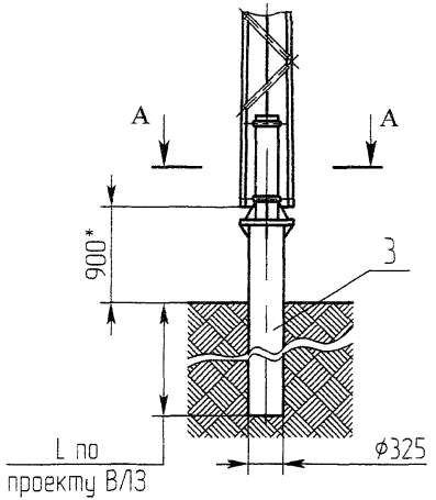
Вариант установки опоры на фундамент ФС10.219/325
