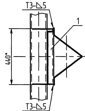
Вид В (лист 1) M1:10
