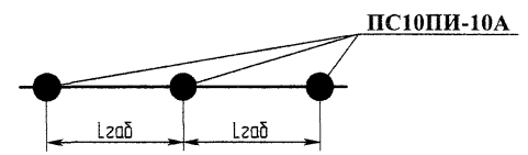
Схема установки опоры на ВЛЗ
