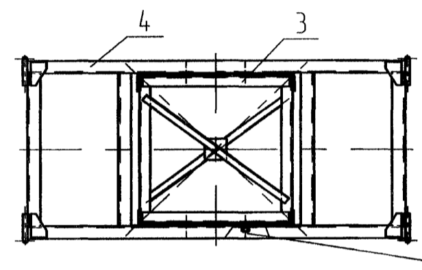
Вид Г подвеска натяжная изолирующая (поз 24) условно не показаны М1:20
