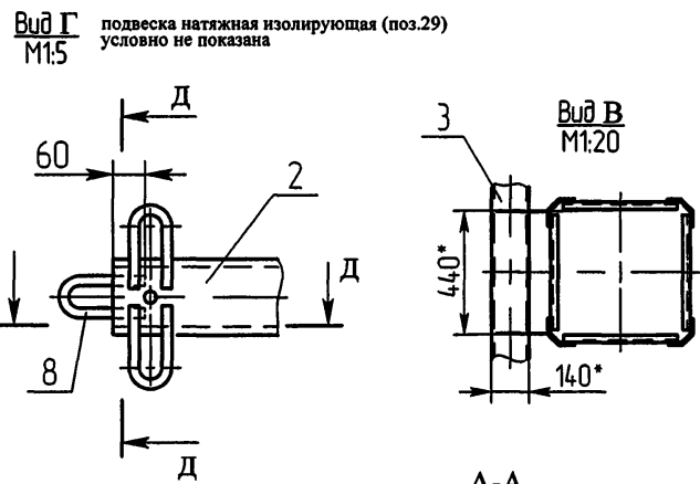
Схема установки опоры на ВЛЗ
