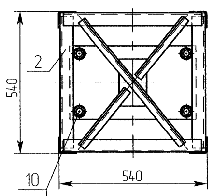
Схема установки опоры на ВЛЗ
