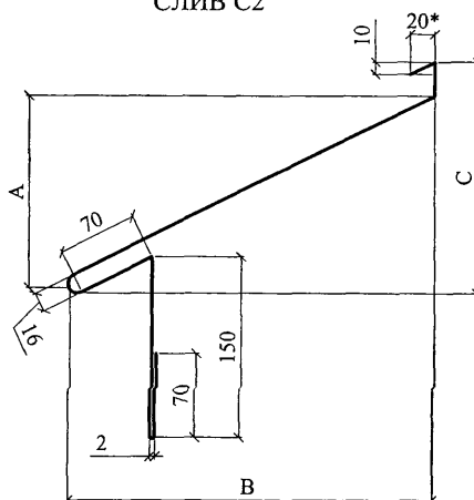
СЛИВ С2
