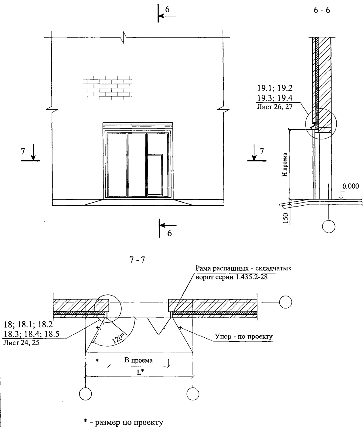
СХЕМА № 5
