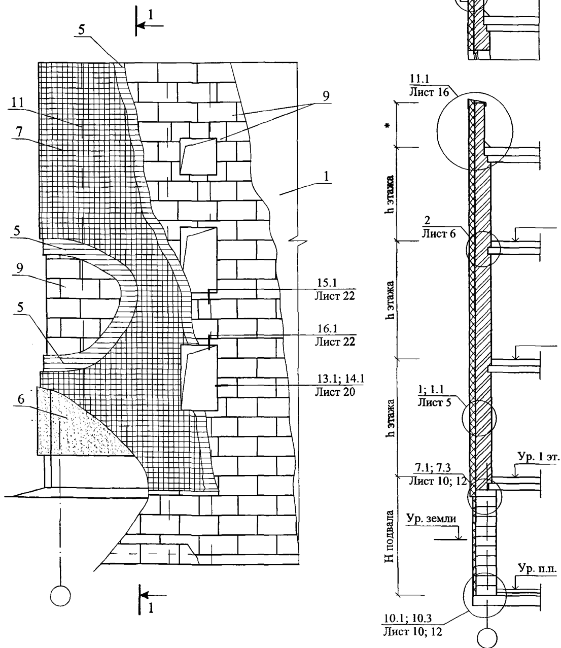
СХЕМА № 1. Расположение минераловатных плит, сетки и штукатурки
