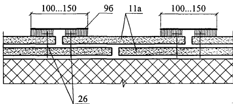
Узел "B.1"
