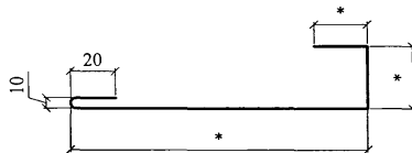
НАЩЕЛЬНИК Н2
