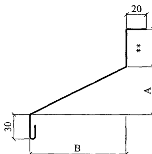
СЛИВ С5
