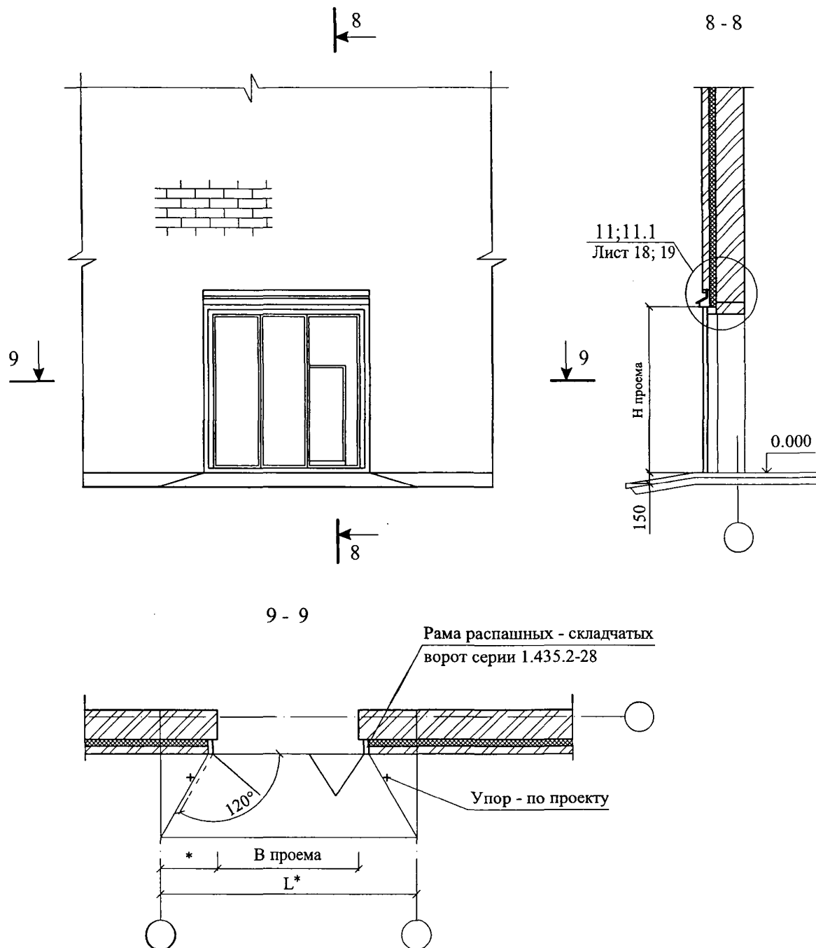
СХЕМА № 5
