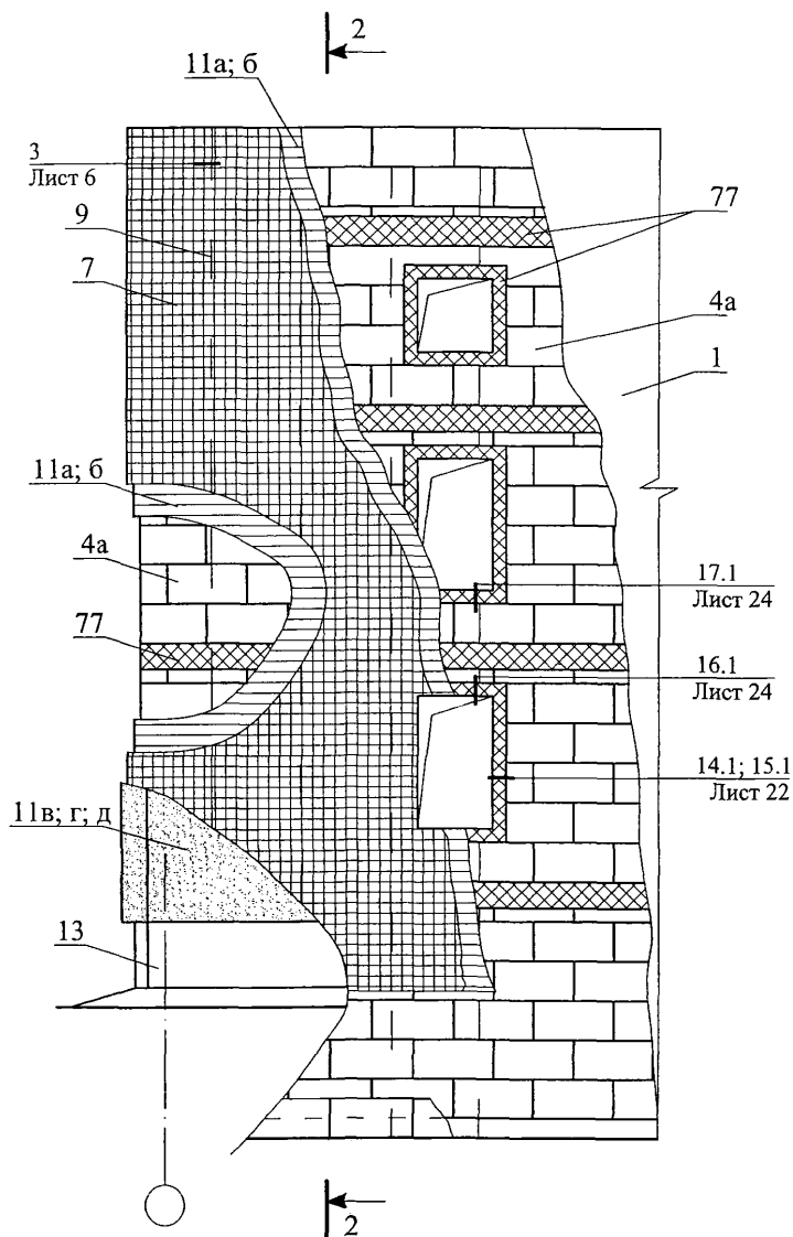
СХЕМА № 2. Расположение плит утеплителя из экструдированного пенополистирола, расщечек, сетки и штукатурки
