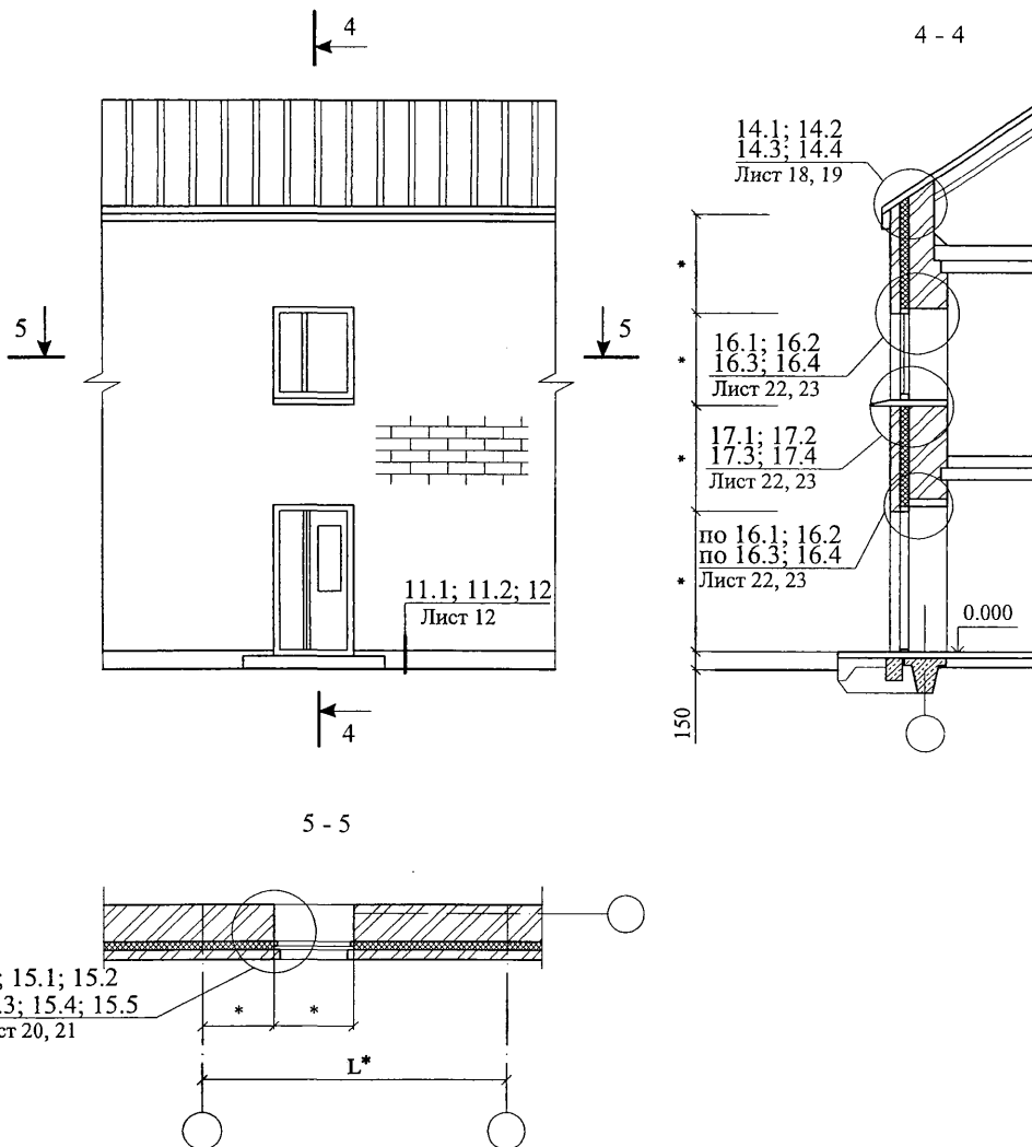
СХЕМА № 4
