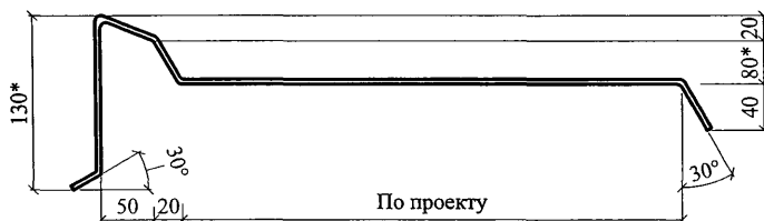
КОСТЫЛЬ К3
