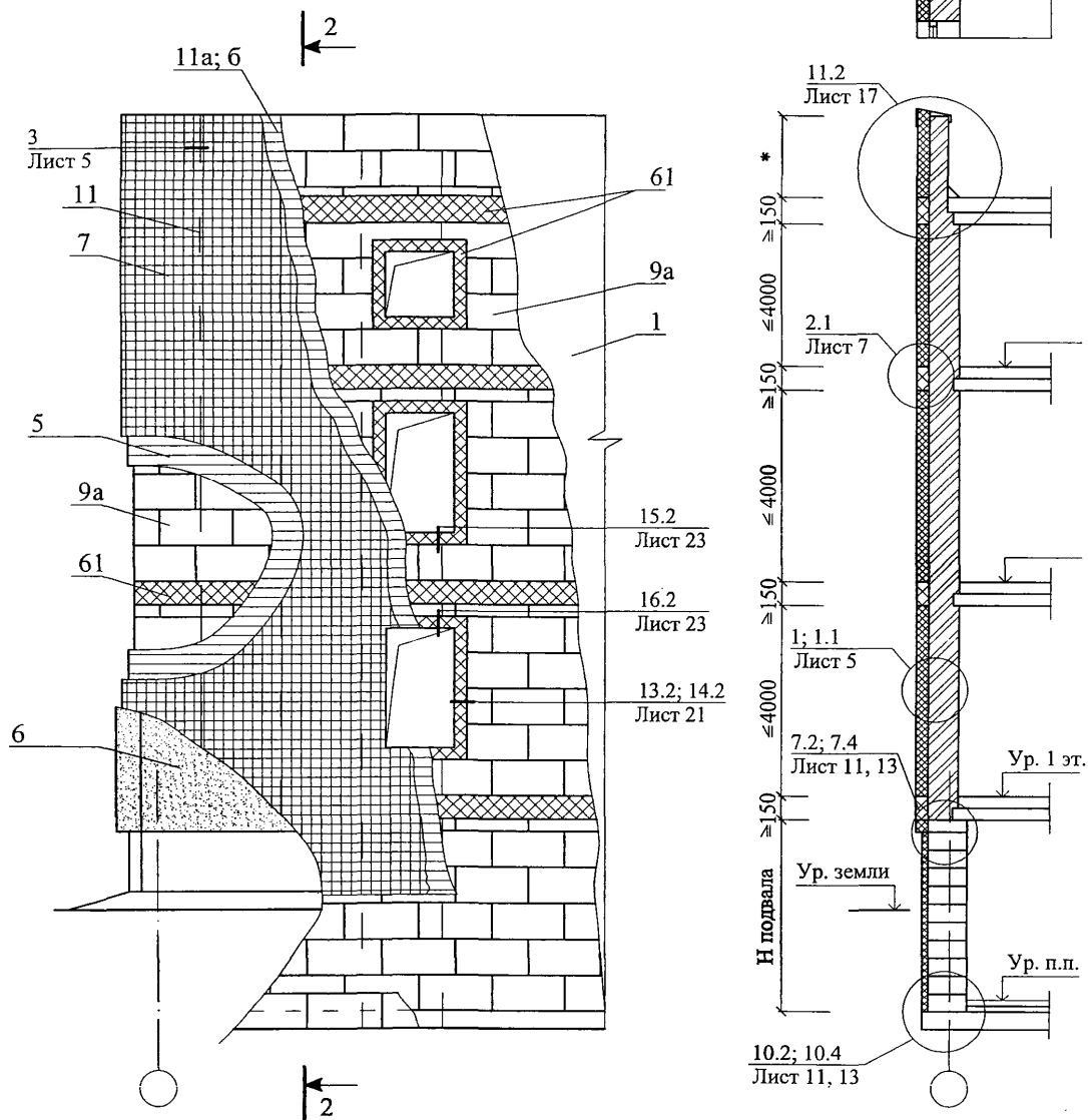
СХЕМА № 2. Расположение плит утеплителя из экструзионного пенополистирола, расщечек, сетки и штукатурки
