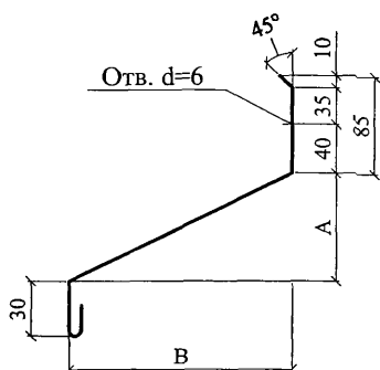
СЛИВ С3
