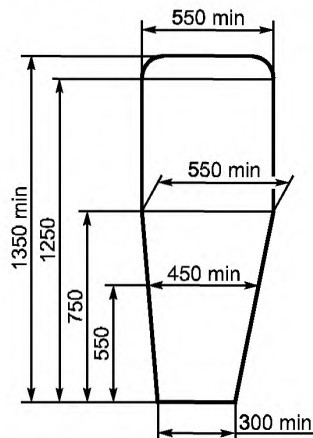
Рисунок 5 — Основные размеры дверного проема
