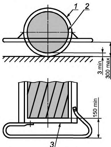
Рисунок 9 — Измельчитель
