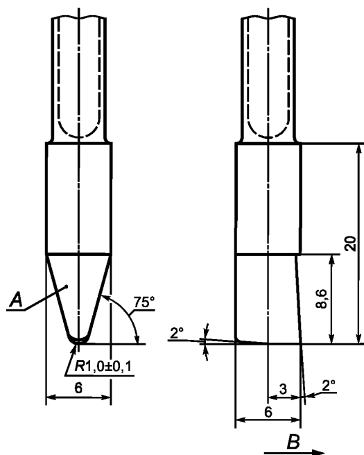
А — твердосплавный наконечник типа К10 по ГОСТ 3882; В — направление движения
