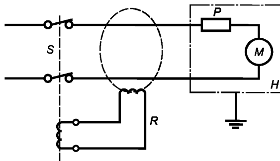
S — источник питания; H — корпус; R — устройство остаточного тока ( I_{\Delta n} = 30 мА); P — устройство тепловой защиты двигателя (наружное или внутреннее), если имеется; M — двигатель
