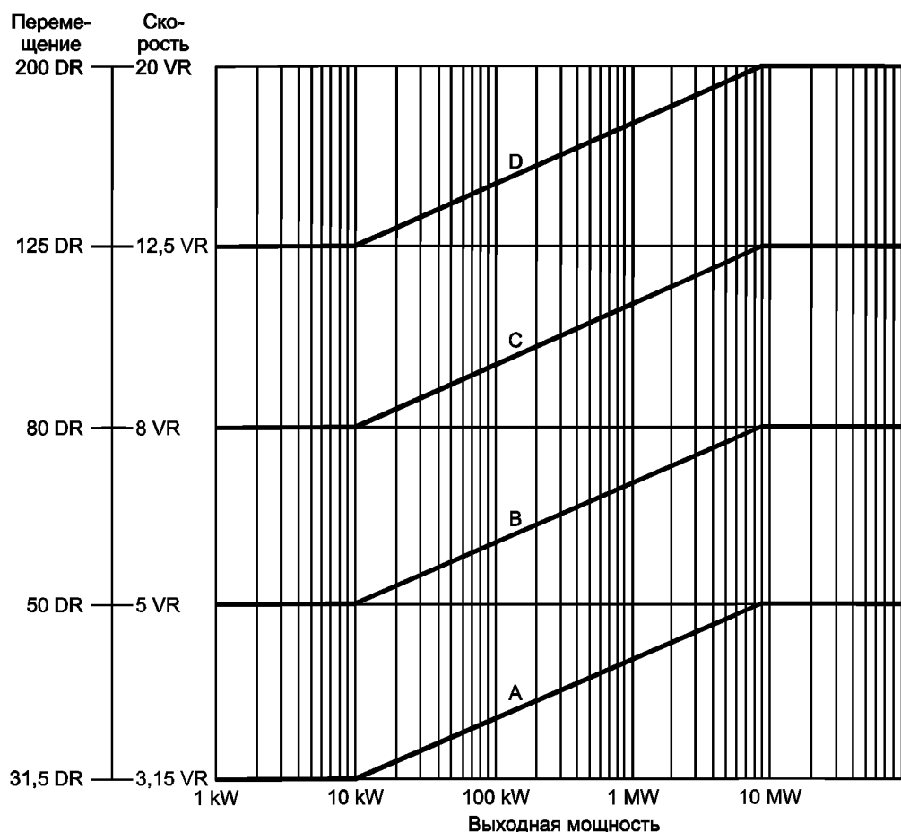
Рисунок С.1 — Ориентировочные классы вибрации
