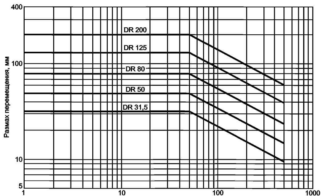
Рисунок 1 — Кривые классов вибрации для вибрации вала
