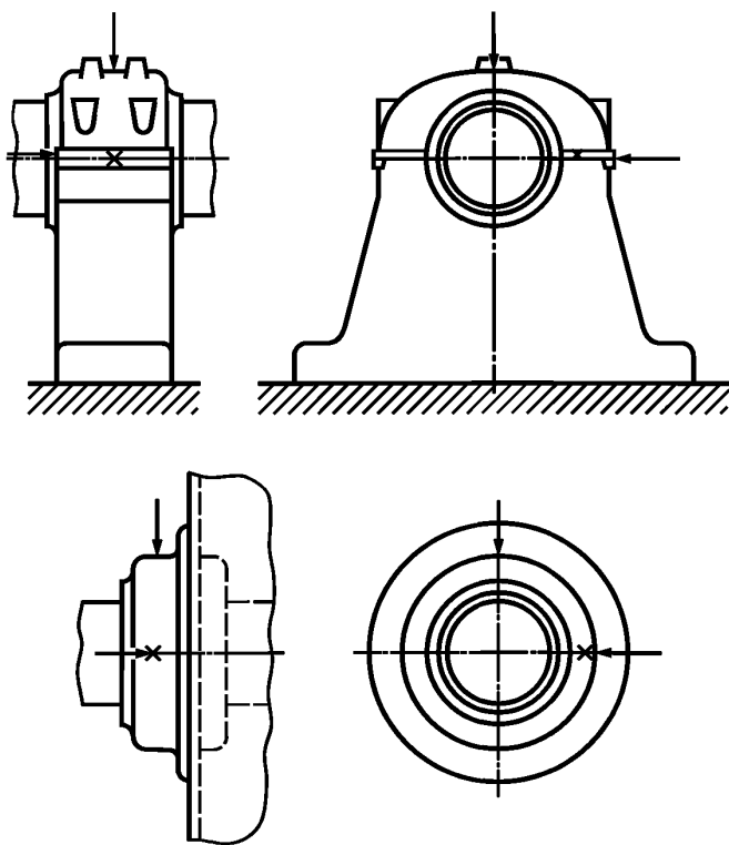
Рисунок 1 — Точки измерений на коренных подшипниках
