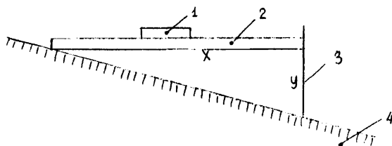
Рис. I. Определение уклона дороги с применением уровня, рейки и линейки:
