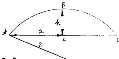
Рис. 2. Схема определения радиуса закругления упрощенным методом
