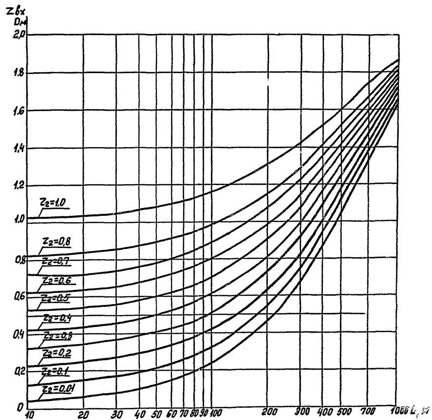
Рис. 10 Значения Z\delta_x = f(L, Z_2) для земли с \rho = 500 \text{ Ом}\cdot\text{м}
