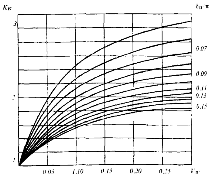
Рис. 3.1.3.2 Коэффициент динамичности ветровых нагрузок
