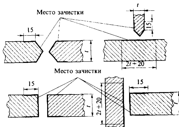
Рис. 2.8.10 Схема зачистки кромок стыкуемых деталей
