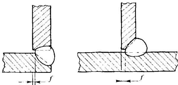
Рис. 2.6.3.4 Примеры односторонних угловых и тавровых соединений с негарантированным полным проваром
