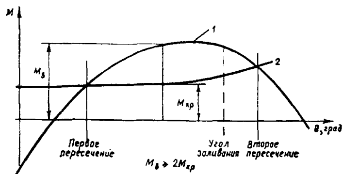
Рис. 2.5.5.4 Кривые восстанавливающего момента (1) и ветрового кренящего (2)
