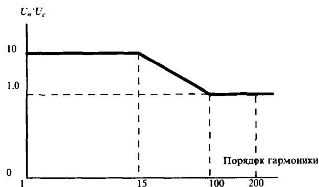
Рис. 2.2.1.2.2 График высших гармоник сети
