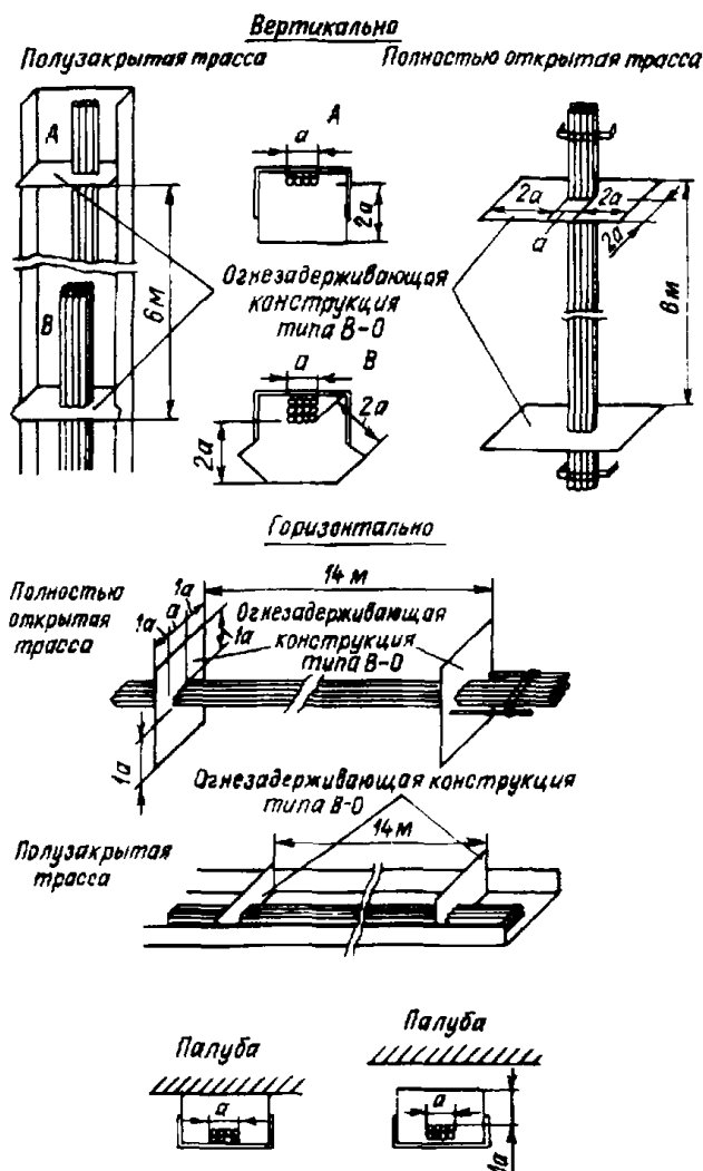
Рис. 16.8.4.3.2-2 Защита кабельных трасс огнезадерживающими конструкциями типа В-0
