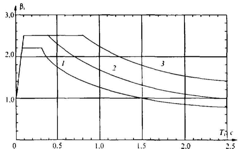
Рис. 3.3.2.4.11 Коэффициенты динамичности \beta(T_i) : кривая 1 — для грунтов I категории; кривая 2 — для грунтов I — II, II, II — III, III категорий при толщине верхнего слоя грунта не более 20 м; кривая 3 — для грунтов I — II, II, II — III, III категорий при толщине верхнего слоя грунта не менее 40 м
