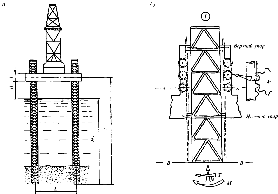
Рис. 3.1.2.1 Идеализация конструкций СПБУ различных уровней: а) конструктивная рама («суперэлемент»), б) расчетный район (I) опорной колонны
