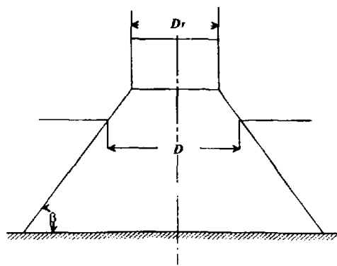
Рис. 3.3.2.3.5-3 Коническая преграда
