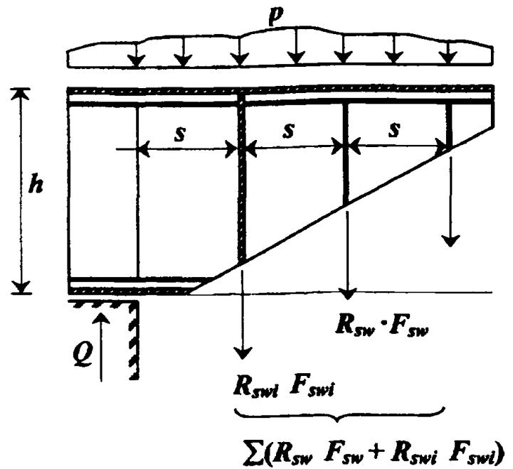
Рис. 3.4.6.3.4 Схема усилий в сечении, наклонном к продоль- ной оси сталежелезобетонного элемента при расчете его прочности на действие поперечной силы
