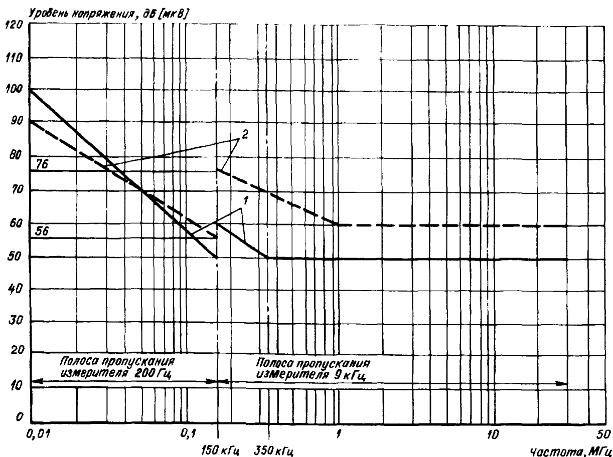
Рис. 2.2.1.4 Допустимые уровни напряжения помех:
