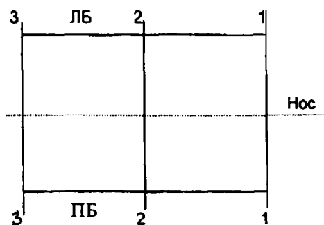
Схема мест (сечений) замеров надводного борта (осадок)
