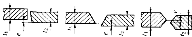
Рис. 2.7.1.11-1 Нарушение соосности деталей для стыковых соединений:
