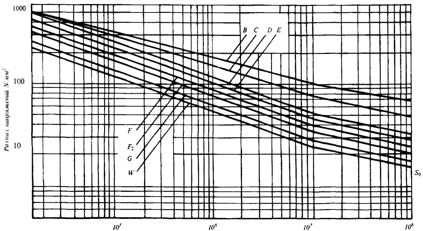
Рис. 2.4.4.8-1 Кривые усталости
