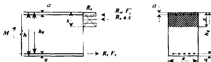
Рис. 3.4.6.2.2-1. Схема усилий в сечении, нормальном к продольной оси изгибаемого железобетонного элемента при расчете его прочности
