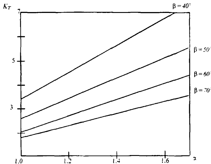
Рис. 3.3.2.3.7 Зависимость коэффициента торосистости K_{\text{Т}} для конических опор от отношения \alpha = h_{\text{конс}}/h_{\text{насл}} и угла конусности \beta
