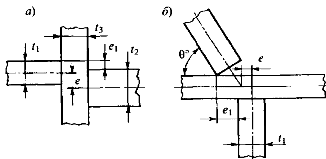
Рис. 2.7.1.11-2 Нарушение соосности деталей для крестообразных соединений:
