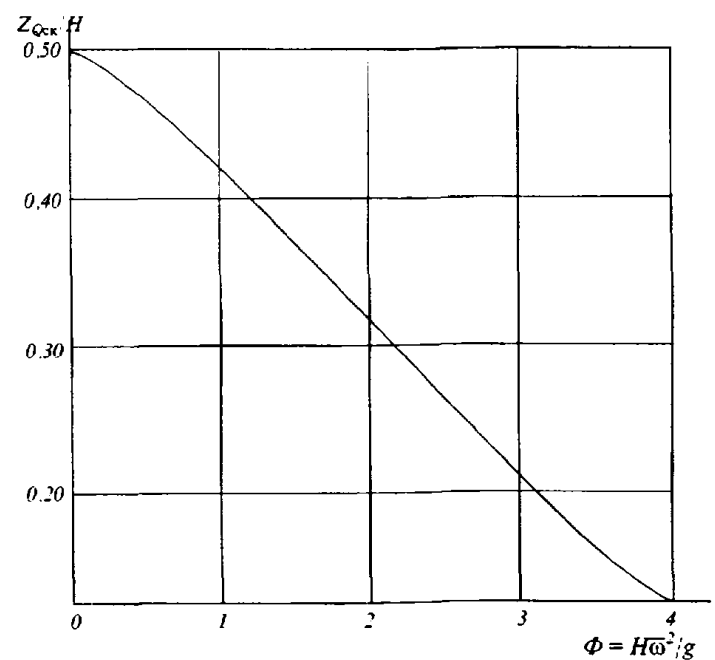
Рис. 3.1.4.13-2 Зависимость Z_{Q_{ск}}/H от параметра \Phi = H\bar{\omega}^2/g
