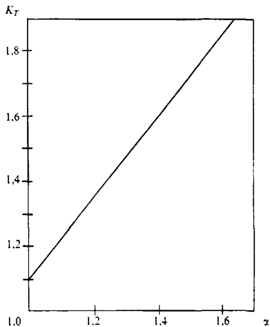
Рис. 3.3.2.3.4 Зависимость коэффициента торосистости K_T для цилиндрических опор в зависимости от \alpha = h_{конс} / h_{насл}
