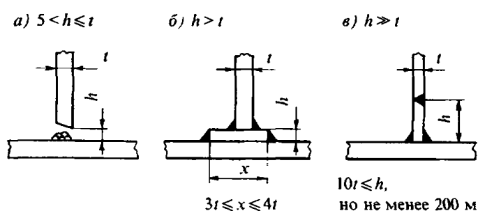
Рис. 2.7.1.10 Схемы устранения недопустимых зазоров для тавровых соединений:
