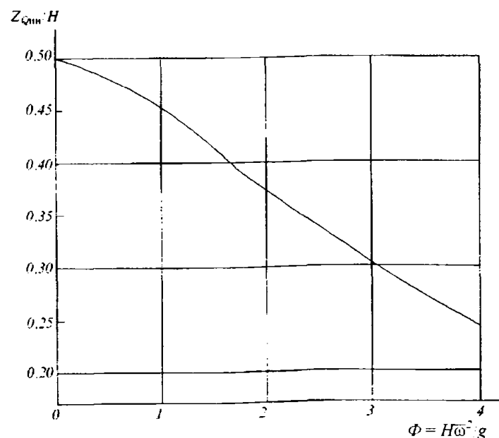
Рис. 3.1.4.13-3 Зависимость Z_{Q_{ин}}/H от параметра \Phi = H\bar{\omega}^2/g
