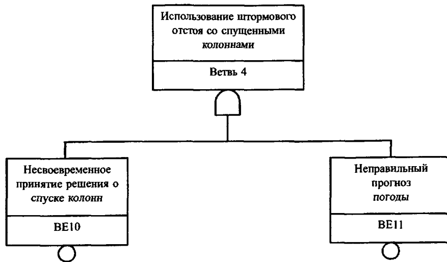
Продолжение построения дерева ошибок и неполадок
