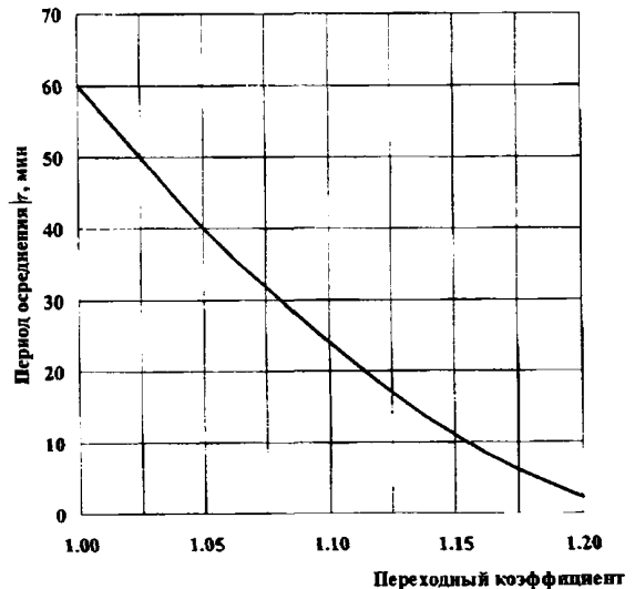
Рис. 2.2.2.4 График переходных коэффициентов v_t/v_{60}
