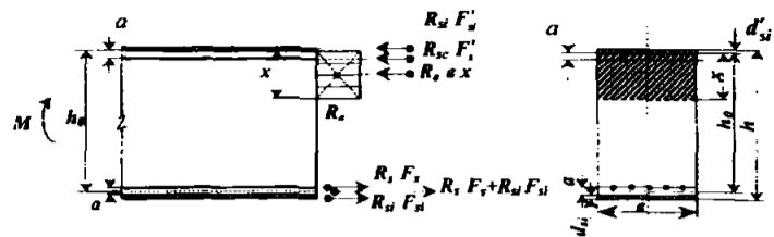
Рис. 3.4.6.2.2-2. Схема усилий в сечении, нормальном к продольной оси изгибаемого сталежелезобетонного элемента при расчете его прочности
