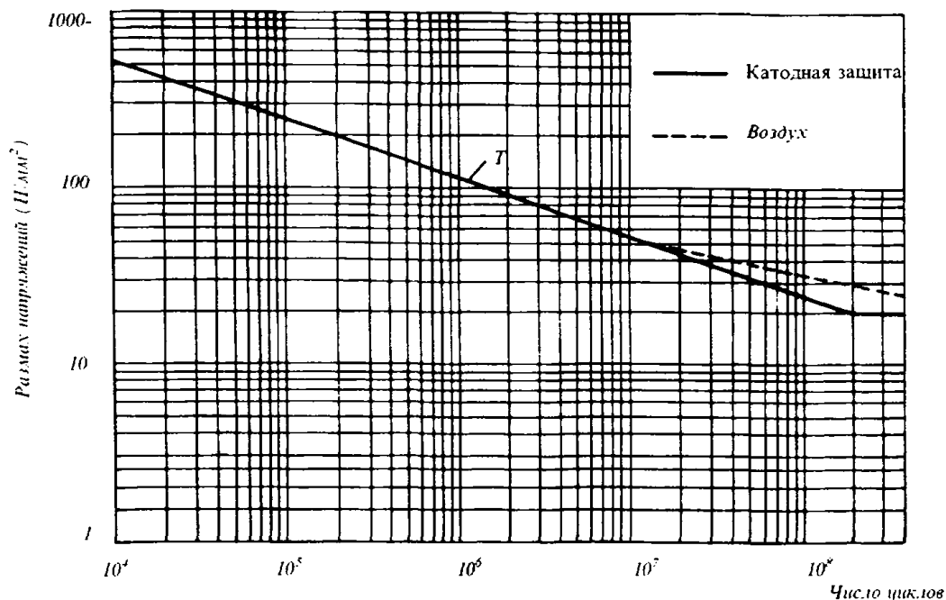
Рис. 2.4.4.8-2 Кривые S-N для трубчатых соединений
