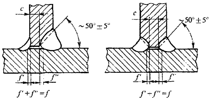
Рис. 2.6.4.1 Примеры двухсторонних тавровых соединений с конструктивным непроваром
