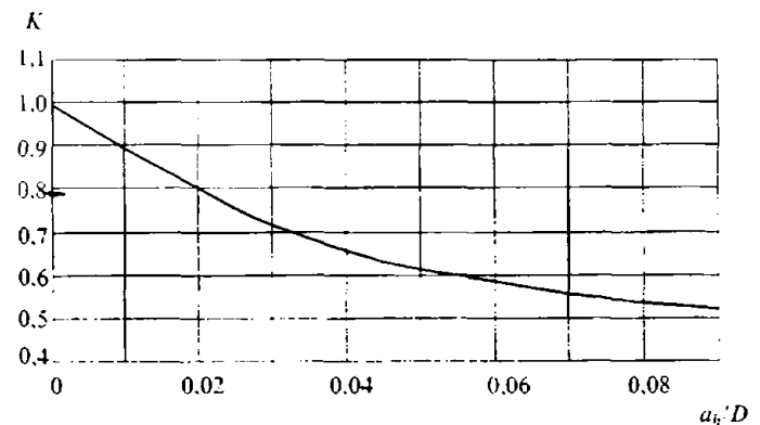
Рис. 3.3.2.3.3-1 Параметр формы K в зависимости от a_h/D
