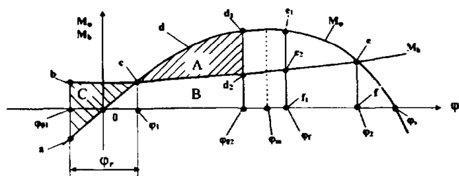
Рис. 3.1.1-1 Диаграмма статической остойчивости с учетом качки:
