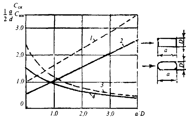
Рис. 3.1.4.1 Коэффициенты скоростного C_{ск} (3, 4) и инерционного C_{ин} (1, 2) сопротивления сечений: — эллиптических (круглых a/D = 1 ); - - - прямоугольных
