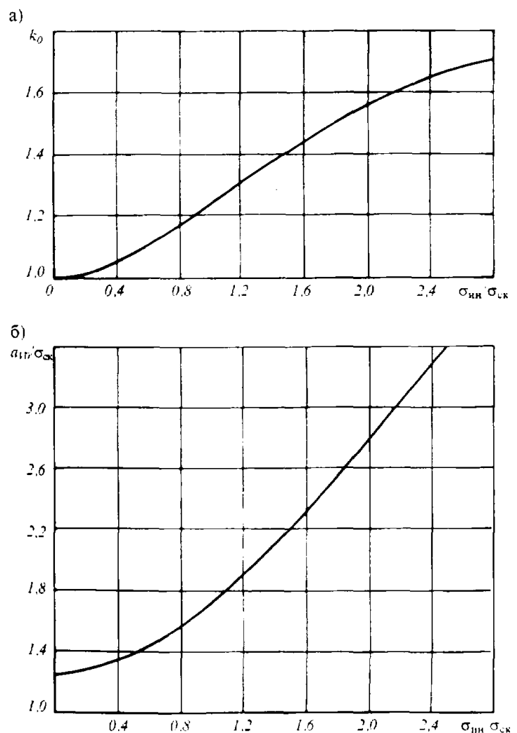
Рис. 3.1.4.9 Зависимость параметров распределения Вейбулла k_0 и a_{10} от соотношения \sigma_{ин}/\sigma_{ск}
