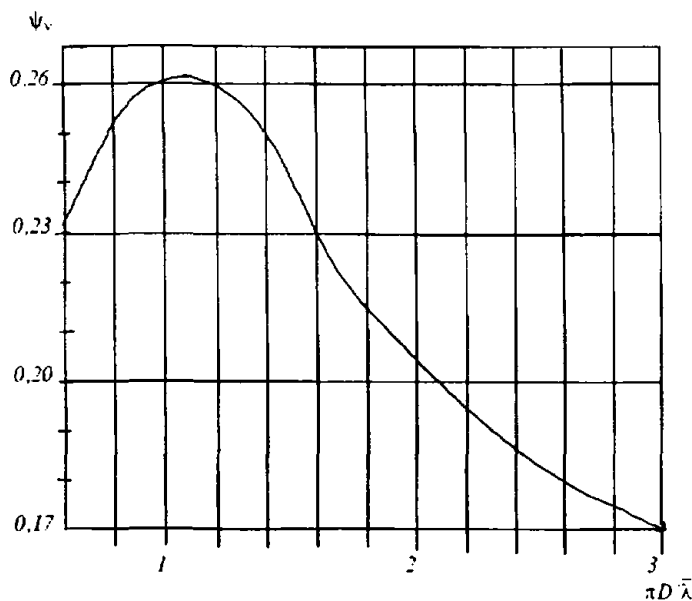
Рис. 3.3.2.1.7 Значение параметра \psi_V дополнительного опрокидывающего момента
