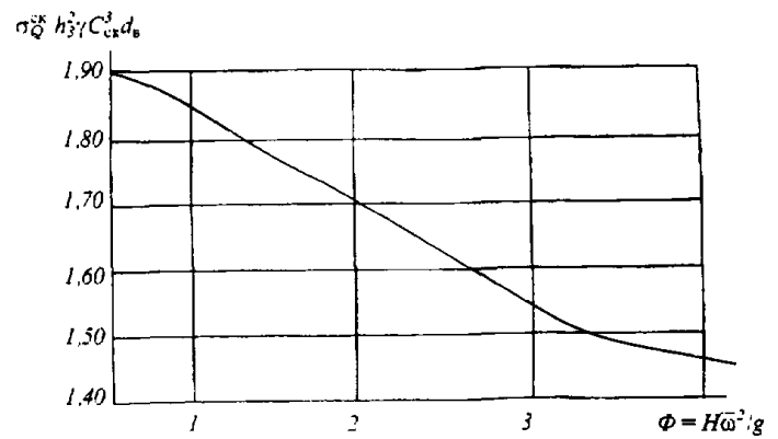
Рис. 3.1.4.13-1 Зависимость \sigma_Q^{ск} h_j^3 \gamma C_{ск}^3 d_b от параметра
