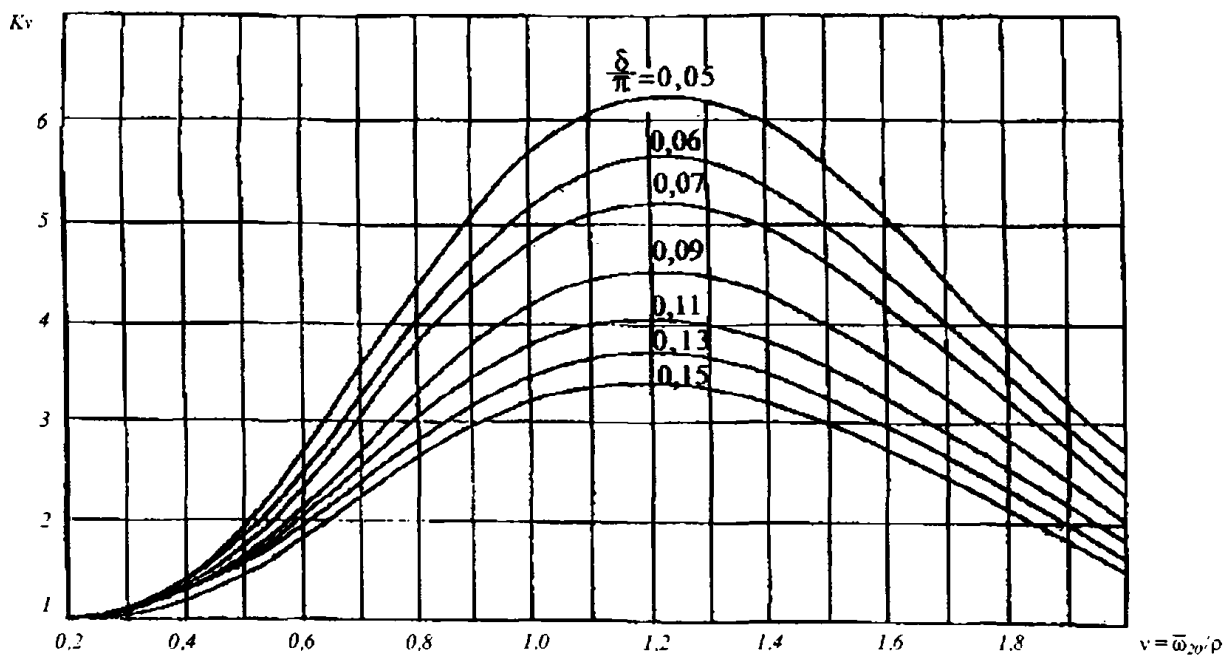
Рис. 3.1.4.3 Коэффициент динамичности скоростной и инерционной составляющих волновой нагрузки
