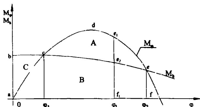
Рис. 3.1.1-2 Диаграмма статической остойчивости без учета качки
