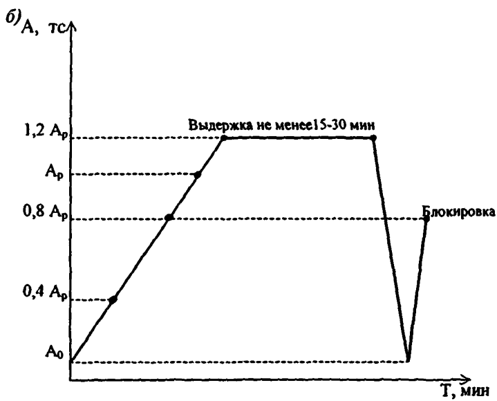
Рис. 5. Программа контрольных (а) и приемочных (б) испытаний
