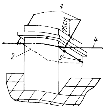
Рис. 19. Крепление молниеприемника к дымовой трубе
