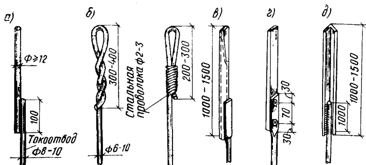
Рис. 8. Конструкции молниеприемников
