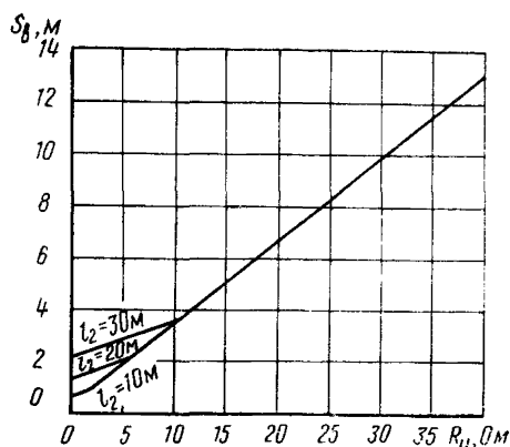
Рис. 7. Наименьшие допустимые расстояния от тросостойки до защищаемого объекта l = 50 \div 200 \text{ м} и l_1 = 40 \text{ м}
