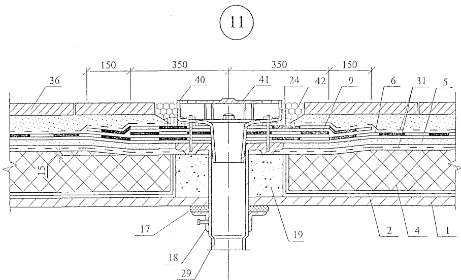
Воронка внутреннего водостока при традиционной эксплуатируемой кровле
