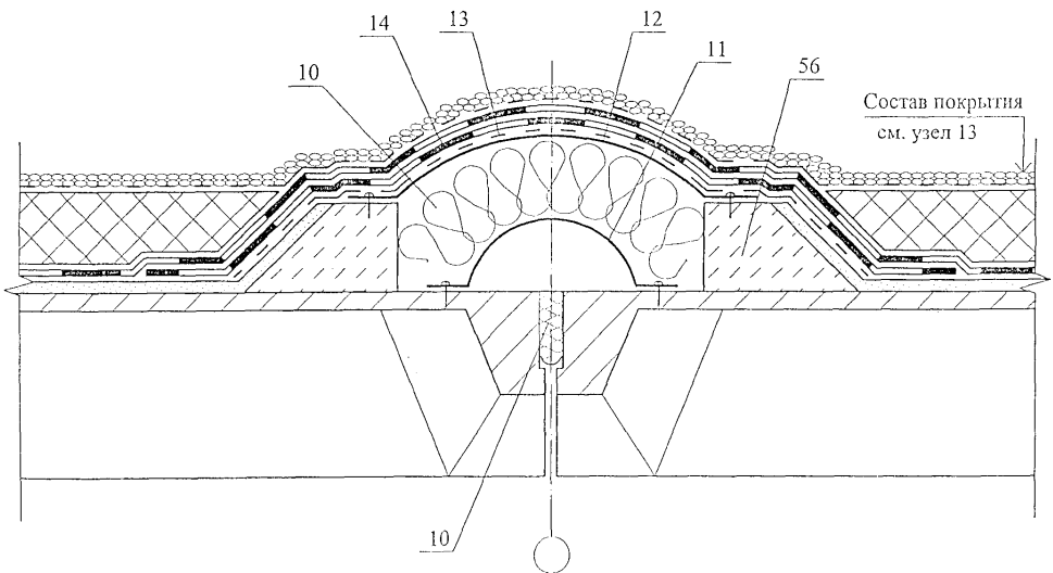
20 Деформационный шов
