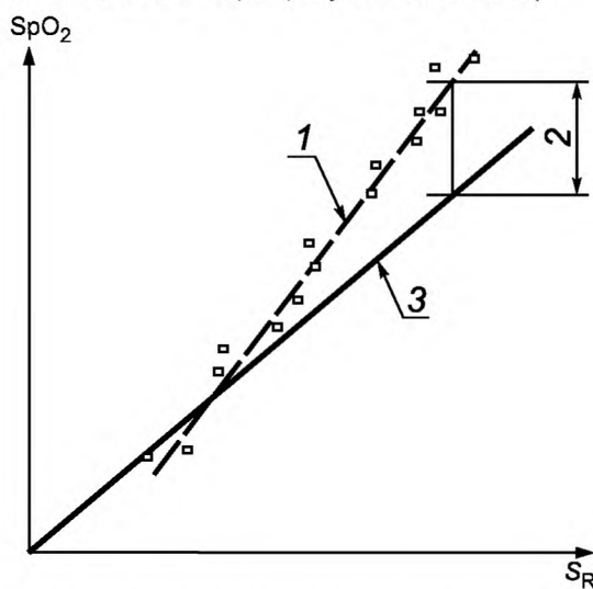
Рисунок СС.4 — Графическое представление определения локальной систематической погрешности (Показания SpO_2 испытуемого датчика в зависимости от показаний S_R эталонного прибора)
