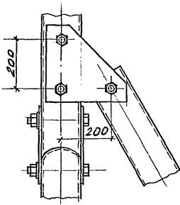
IV M1:10
