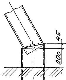
III M 1:10
