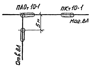
Схема установки опор
