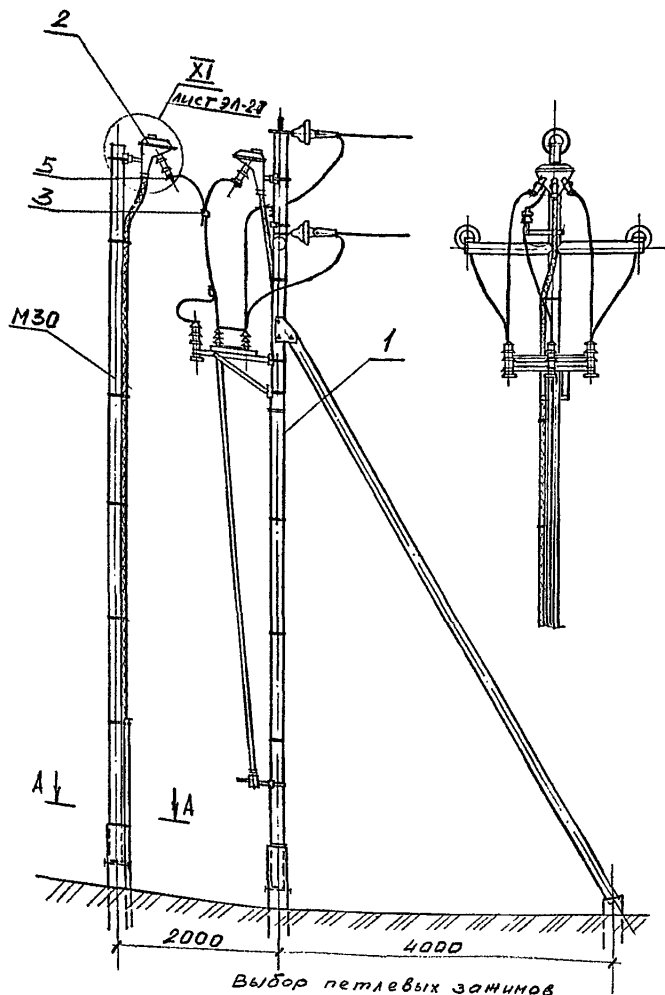
Выбор петлевых зажимов
