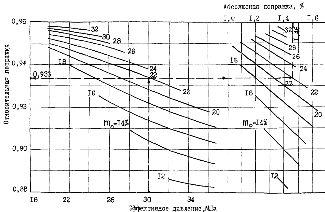
Номограмма для определения термобарических поправок к коэффициенту пористости
