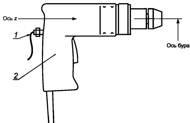
1 — датчик вибрации; 2 — основная рукоятка
