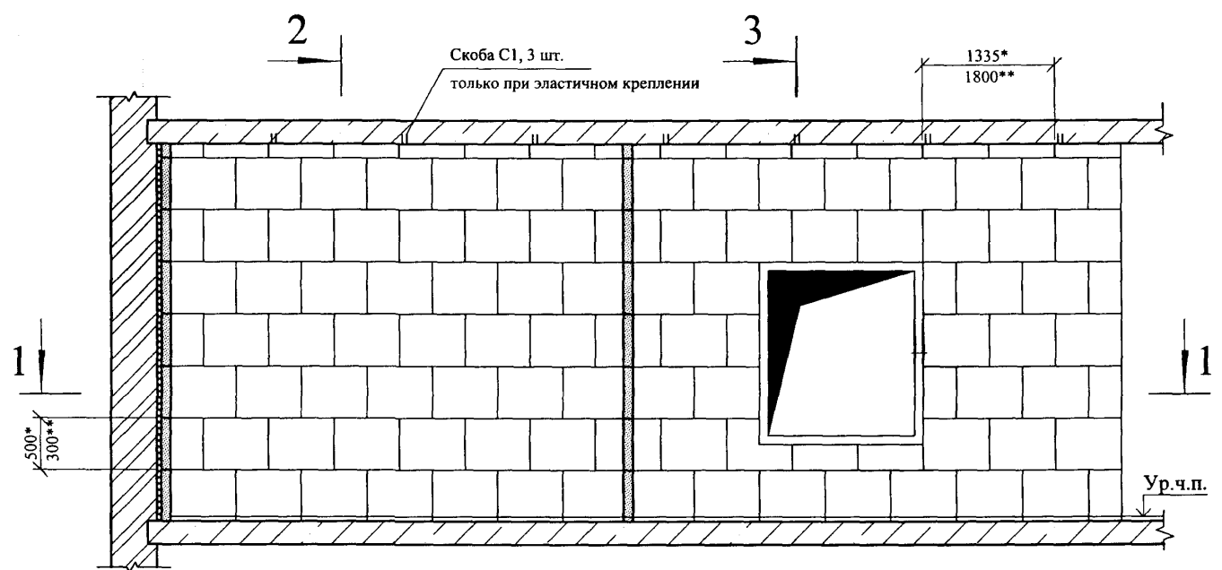
Схема облицовки стен
